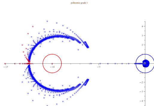
(b) Conjunto de ceros de \varphi_0, \dots, \varphi_{70} .
