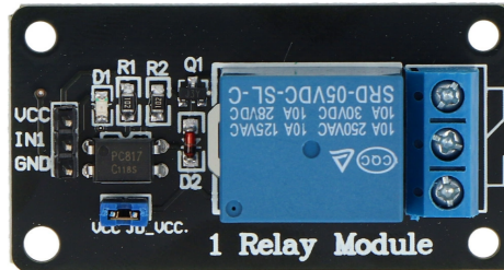
Rysunek 4: Moduł przekaźnika.
