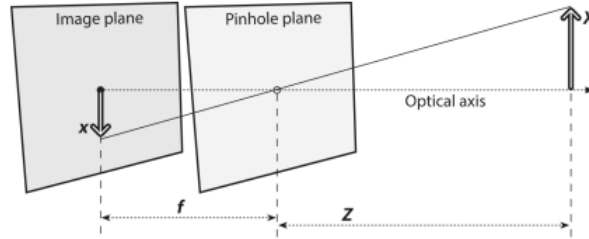
Rysunek 7: Model kamery otworkowej
