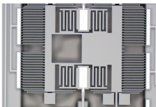
(a) Microscopia de um acelerômetro MEMS capacitivo [2].
