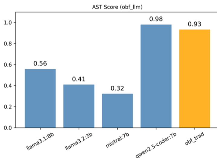
Ilustración 22. AST Score en la ofuscación
