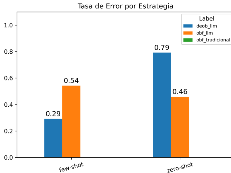
Ilustración 28. Tasa de error por estrategia
