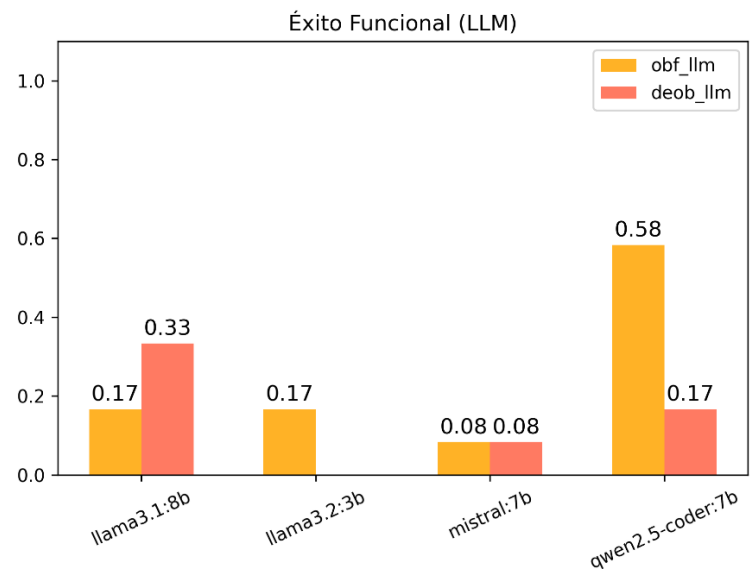
Ilustración 26. Éxito funcional por estrategia
