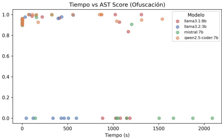
Ilustración 30. Mapa tiempo de ejecución/AST score
