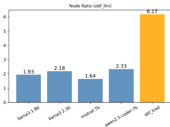
Ilustración 23. Node ratio en la ofuscación
