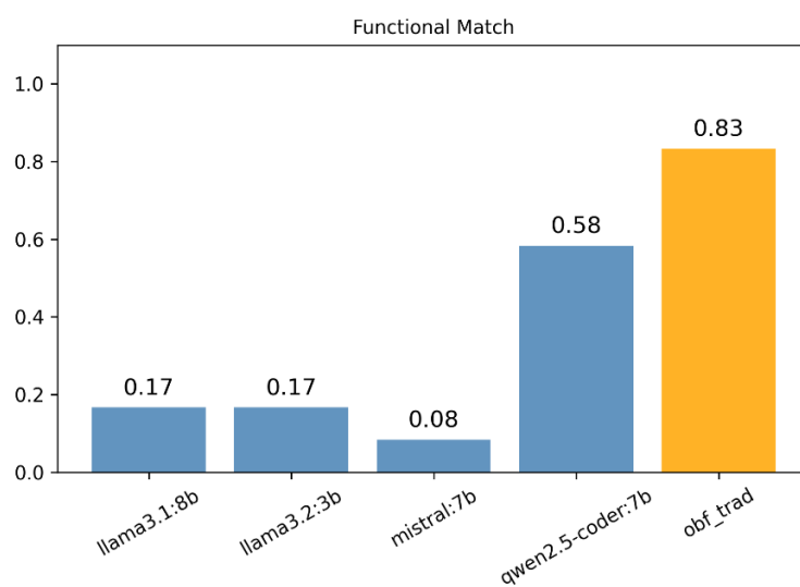
Ilustración 24. Functional match en la ofuscación
