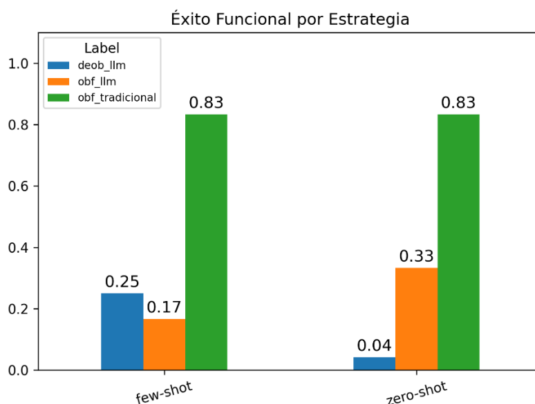
Ilustración 27. Éxito funcional por estrategia
