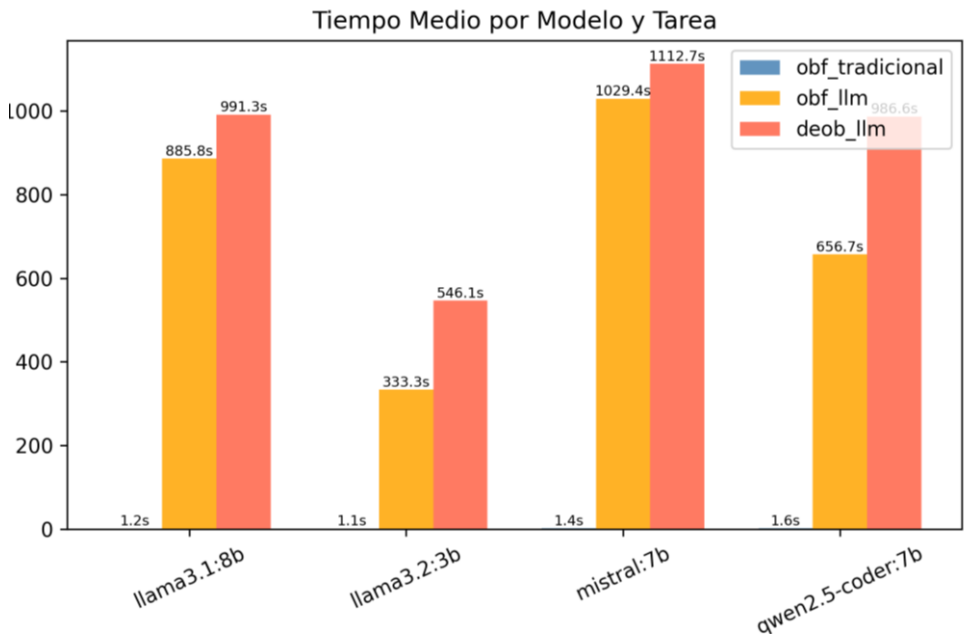
Ilustración 29. Tiempo medio por modelo y tarea
