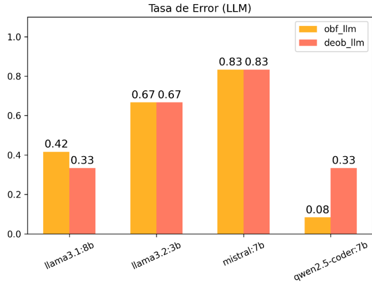
Ilustración 25. Tasa de error por estrategia
