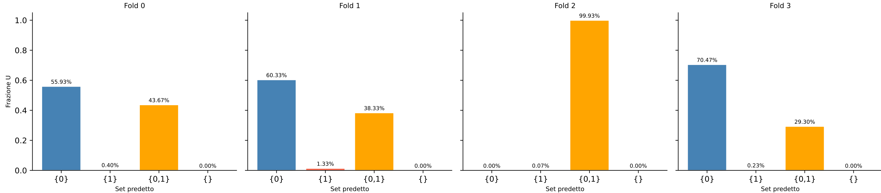
Distribuzione prediction set su U — re_lgbm M3
