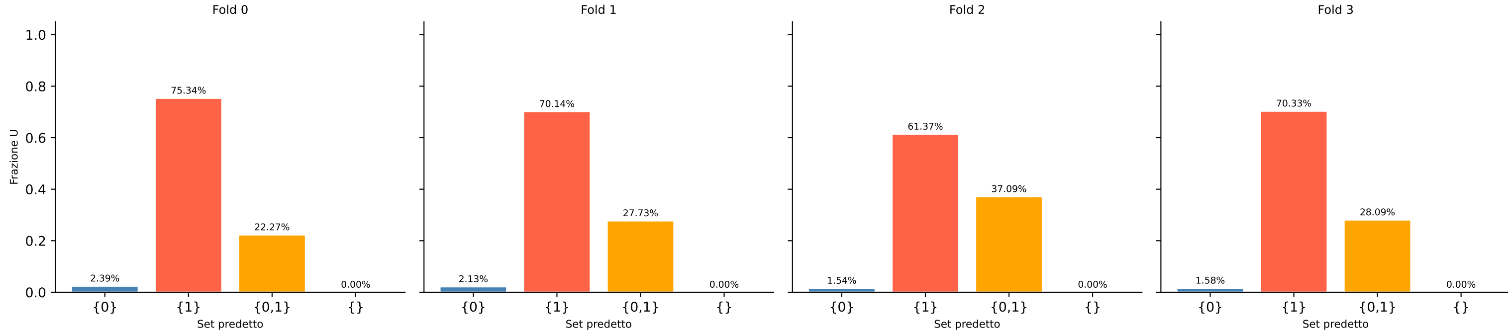
Distribuzione prediction set su U — lgb_supervised M1
