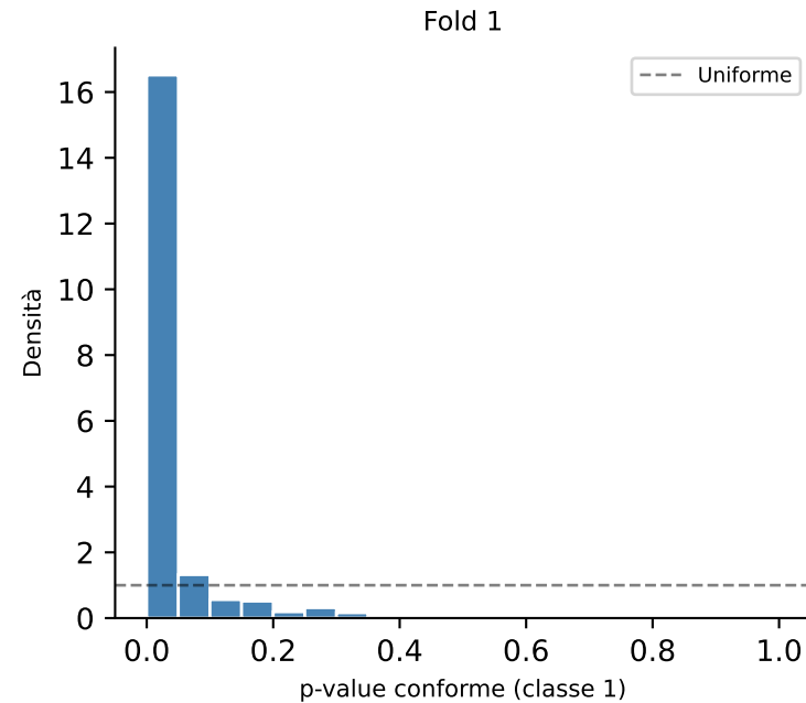
P-value conformi su U (classe 1) — bagging_lgbm M1 Uniforme = nessun segnale; concentrata vicino a 0 = segnale forte
