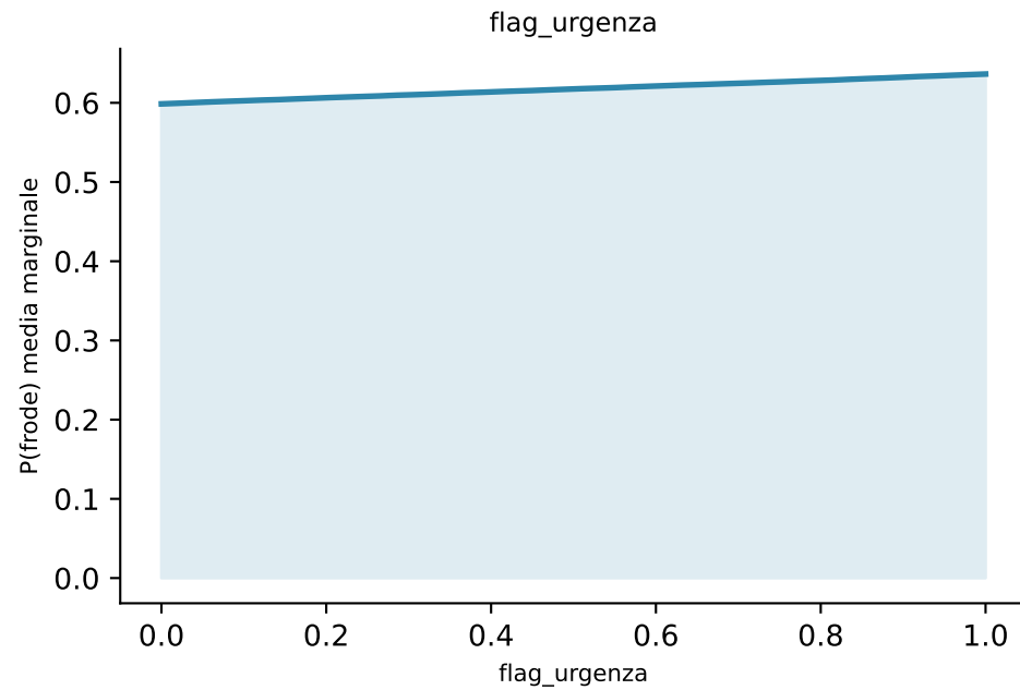
PDP top-3 feature — puet M1 (media marginale, score grezzo pre-Platt)
