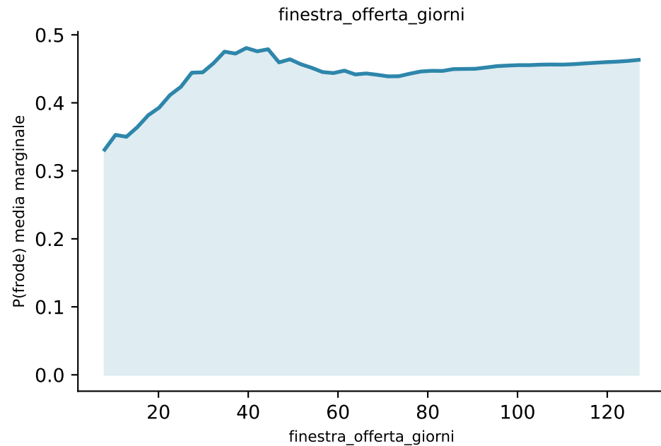
PDP top-3 feature — puet M2 (media marginale, score grezzo pre-Platt)
