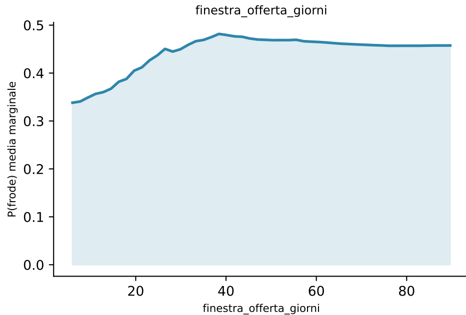
PDP top-3 feature — puet M3 (media marginale, score grezzo pre-Platt)
