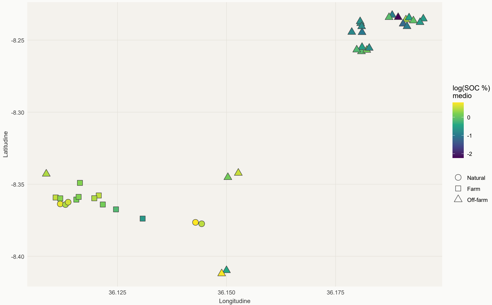
Distribuzione spaziale dei 40 campi
