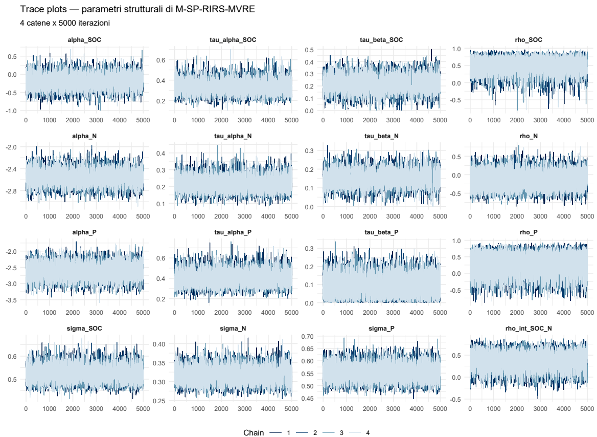
Figura 6: Trace plot delle 4 catene MCMC per \alpha_r , \tau_{\alpha,r} , \tau_{\beta,r} , \rho_r , \sigma_r e \rho_{\text{int}}(\text{SOC}, N) (modello M-SP-RIRS-MVRE, 16 parametri strutturali). Buona mescolanza: nessuna evidenza di mancata convergenza o pattern sistematici.
