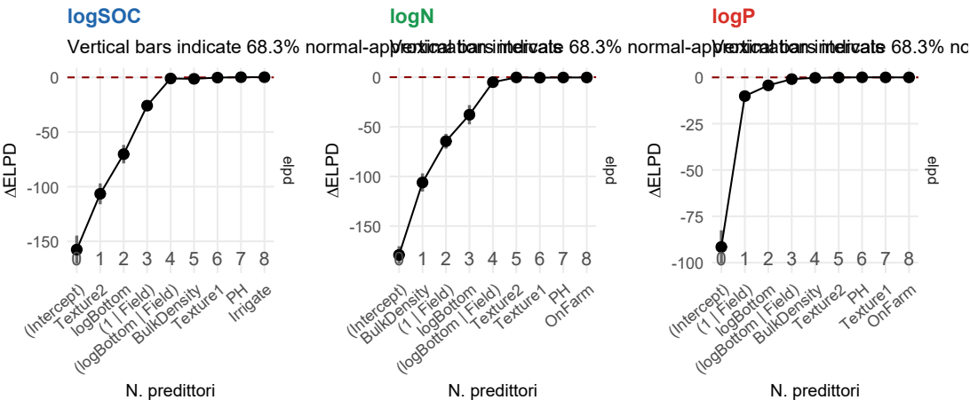
Figura 4: Percorso di selezione projpred per SOC, N e P ( \Delta\text{ELPD} in funzione del numero di predittori; linea tratteggiata: soglia di accettazione \alpha = 0.10 ).
