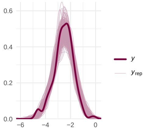
PPC — logP
