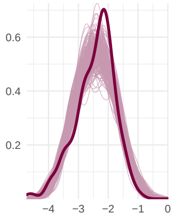
PPC — logN
