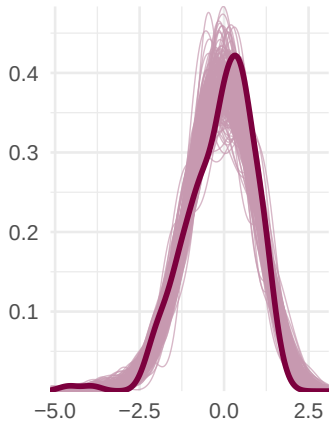
PPC — logSOC
