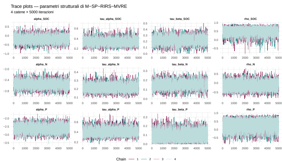
Figura 5: Trace plot delle 4 catene MCMC per \alpha_r , \tau_{\alpha,r} , \tau_{\beta,r} , \rho_r (modello M-SP-RIRS-MVRE). Buona mescolanza: nessuna evidenza di mancata convergenza.
