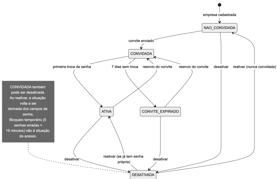
Figura 26 – Diagrama de estados – situação de acesso da empresa
