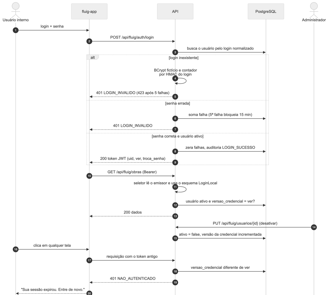
Figura 22 – Diagrama de sequência – login próprio com revogação por versão da credencial
