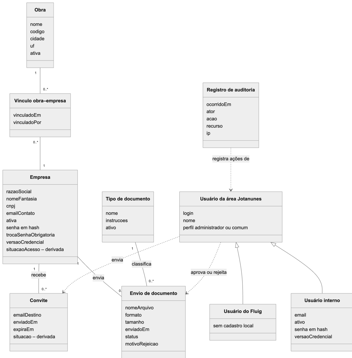
Figura 19 – Modelo do domínio (modelo conceitual)
