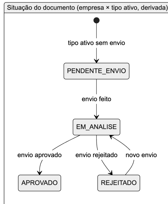
Figura 25 – Diagrama de estados – envio de documento e situação do documento
