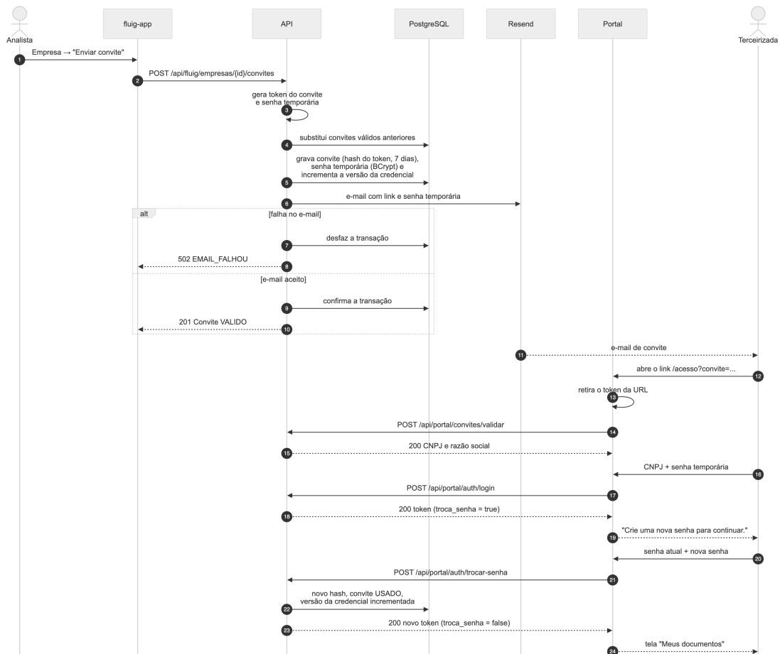
Figura 20 – Diagrama de sequência – convite, e-mail, primeiro acesso e troca de senha
