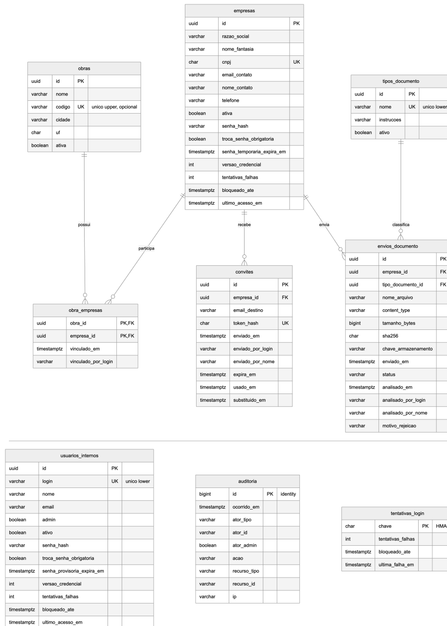
Figura 1 – Modelo lógico do banco de dados
