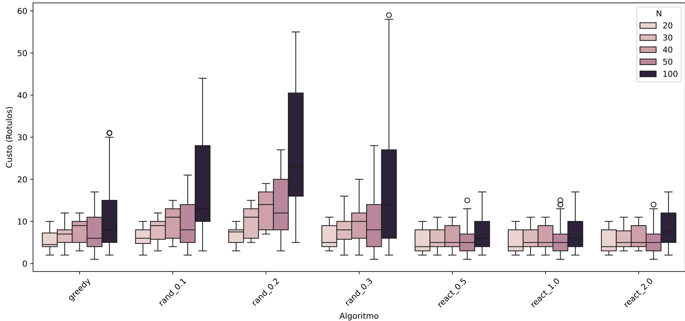
Distribuição de Rotulos Usados ( N \leq 100 )
