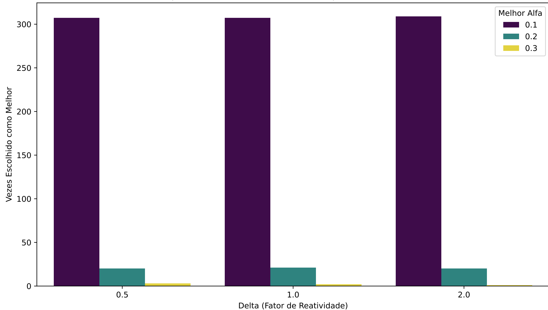
Frequência de Escolha do Melhor Alfa por Delta (N <= 100)
