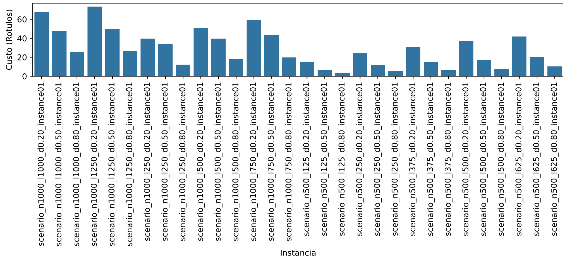
Custo do Guloso (N &gt;= 500)
