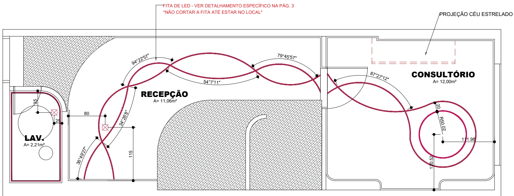
PLANTA BAIXA - LUMINOTÉCNICO ESCALA 1:100
