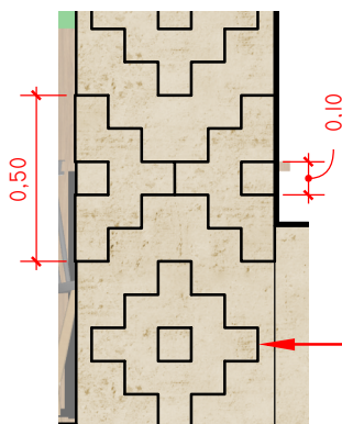
DETALHE MONOLITOS CHAKANA ESC: 1:25
