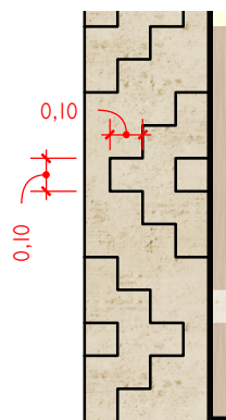
DETALHE MONOLITOS CHAKANA ESC: 1:25
