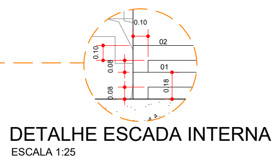
DETALHE ESCADA INTERNA ESCALA 1:25
