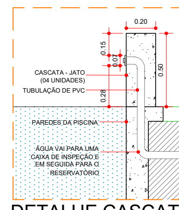
DETALHE CASCATAS ESCALA 1:25
