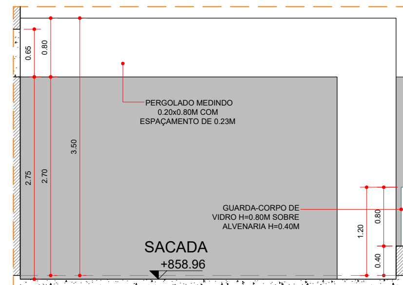
DETALHE PERGOLADO SACADA SUÍTE CASAL ESCALA 1:50
