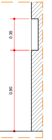
DETALHE NICHOS TODOS OS BANHEIROS ESCALA 1:25
