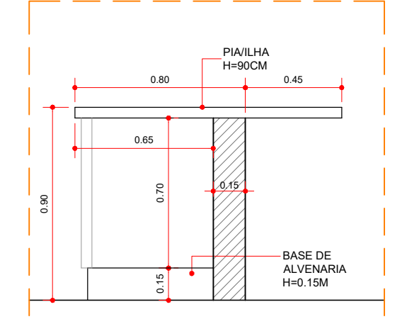
DETALHE DA PIA COZINHA ESCALA 1:25
