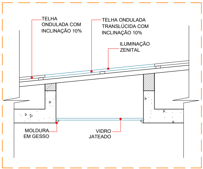
DETALHE ILUMINAÇÃO ZENITAL ESCALA 1:25
