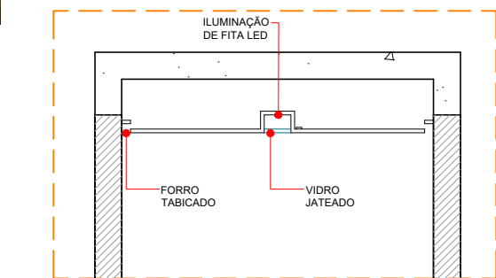
DETALHE RASGO COM ILUMINAÇÃO DE LED E VIDRO JATEADO OU CANALETA DE LED EMBUTIDA NO FORRO DE GESSO ESCALA 1:25
