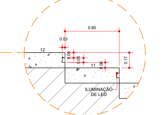
DETALHE ESCADA FACHADA ESCALA 1:25
