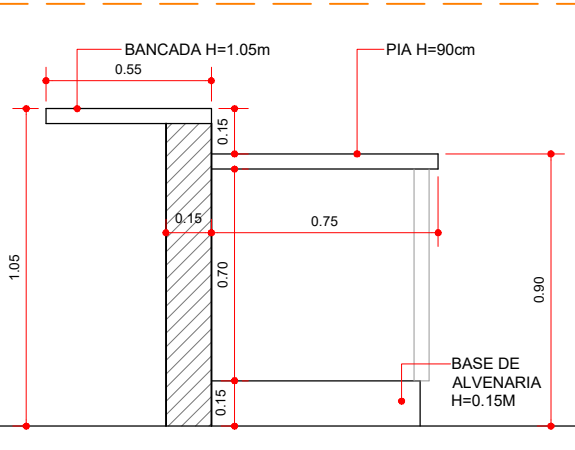
DET. PIA/BANCADA GOURMET ESCALA 1:25
