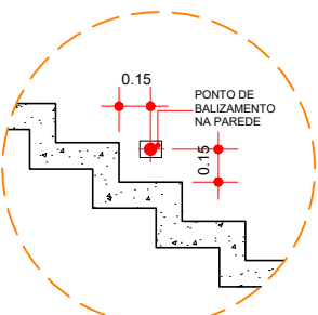
DETALHE ILUMINAÇÃO NA ESCADA ESCALA 1:25
