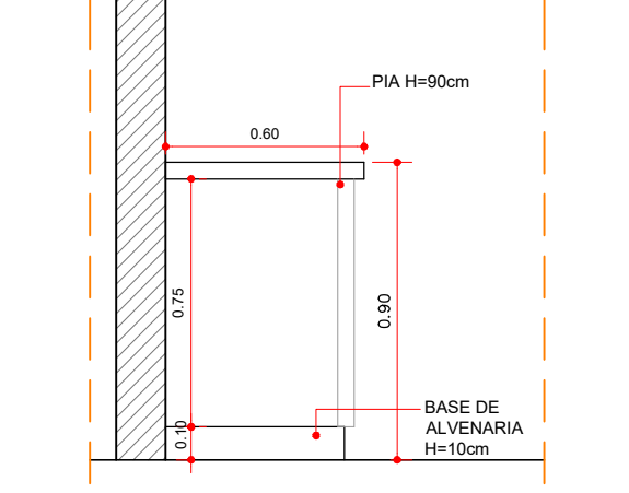
DETALHE DA PIA ESCALA 1:25
