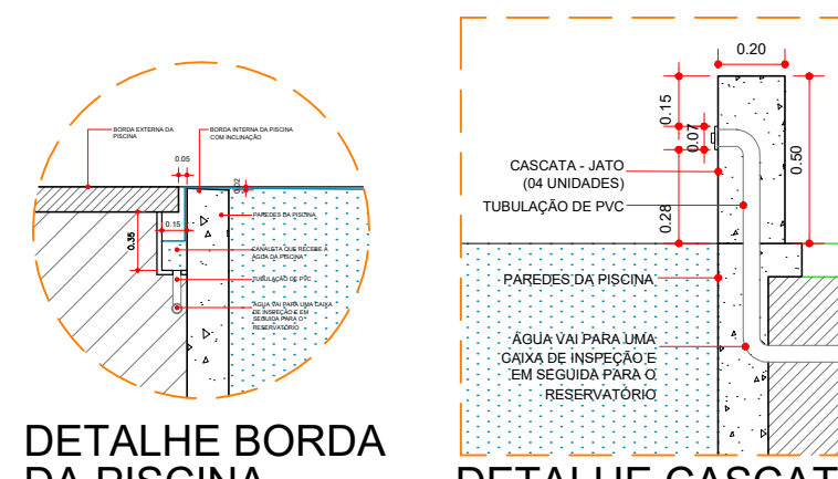
DETALHE BORDA DA PISCINA ESCALA 1:25
