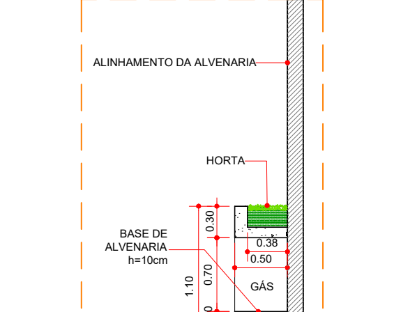
DET. ARMÁRIO DE GÁS ESCALA 1:50
