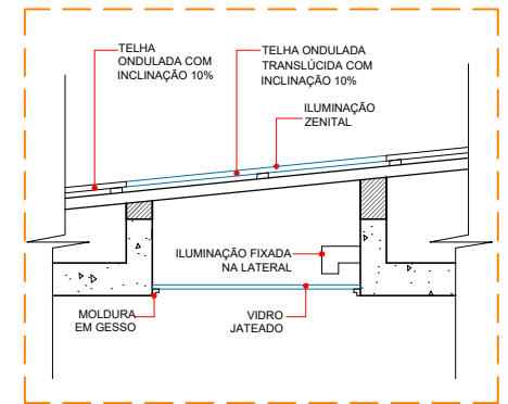
DETALHE DA ILUMINAÇÃO ZENITAL ESCALA 1:25
