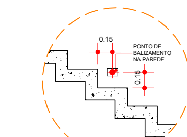
DETALHE ILUMINAÇÃO NA ESCADA ESCALA 1:25
