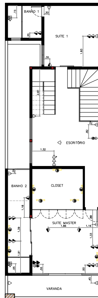
PAVIMENTO SUPERIOR
