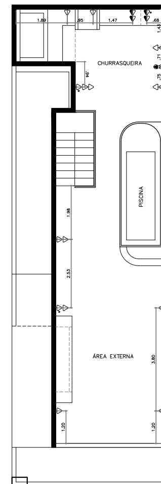
2º PAVIMENTO SUPERIOR (NOVO)
