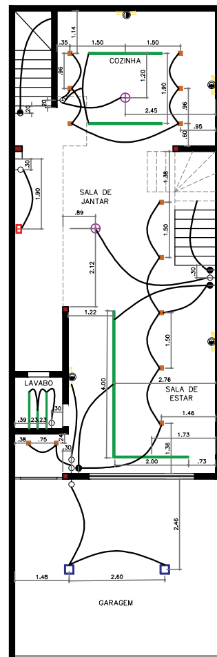
PAVIMENTO TÉRREO
