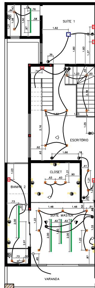
PAVIMENTO SUPERIOR
