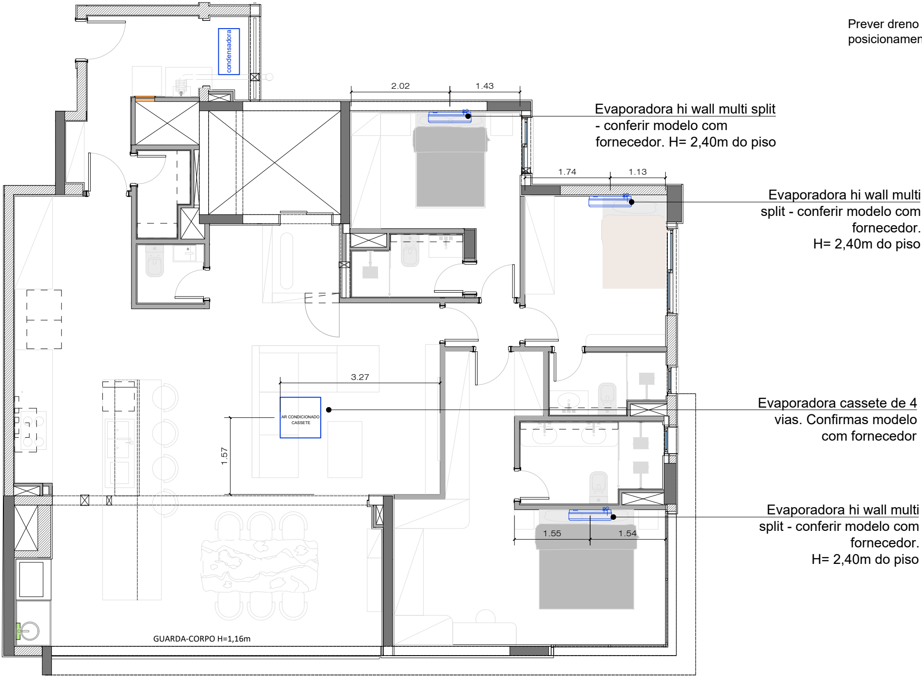
PLANTA DE AR CONDICIONADO ESCALA 1:75
