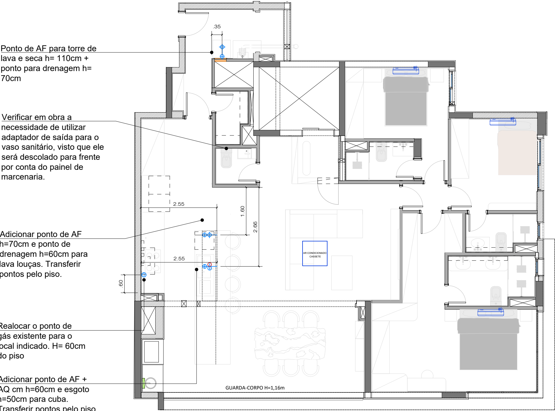
PLANTA DE HIDRÁULICA E GÁS ESCALA 1:75
