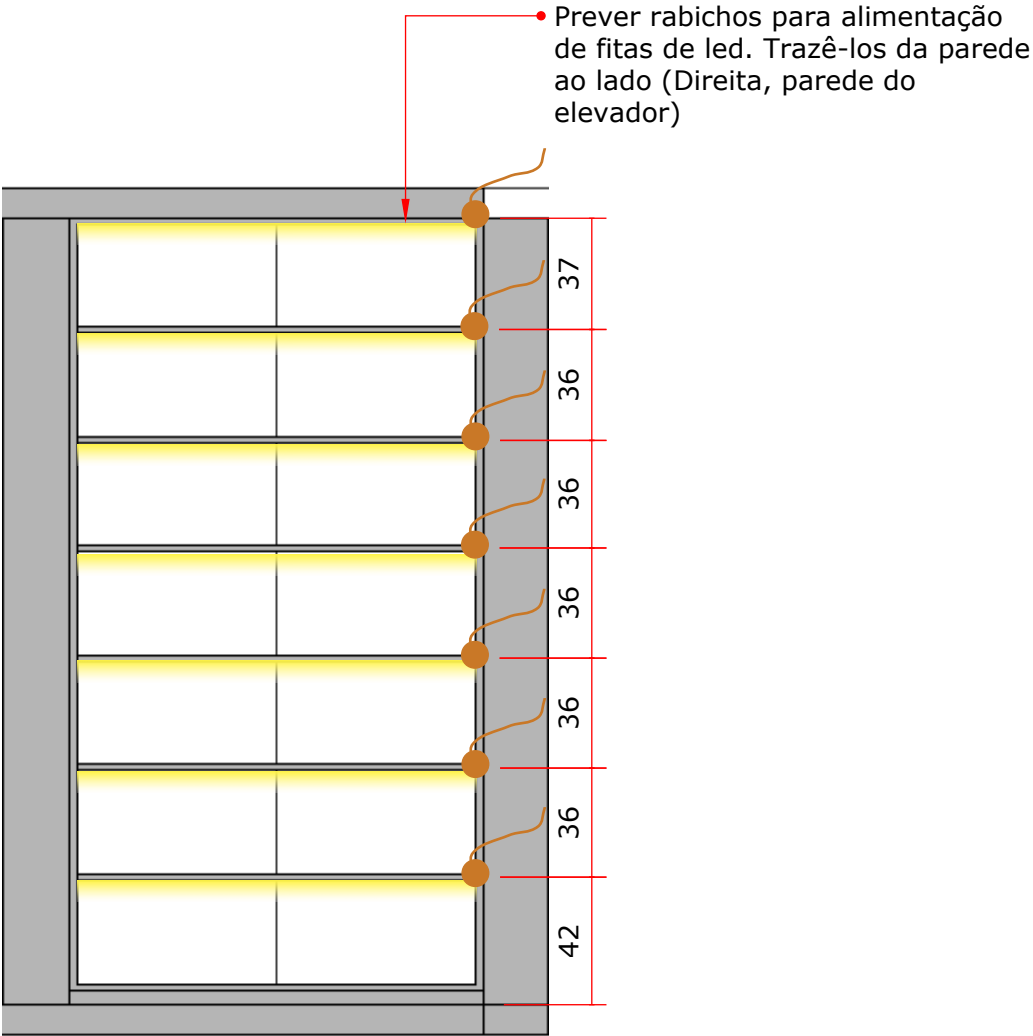
VISTA 5 - PONTOS ELÉTRICOS HALL ESCALA 1:25
