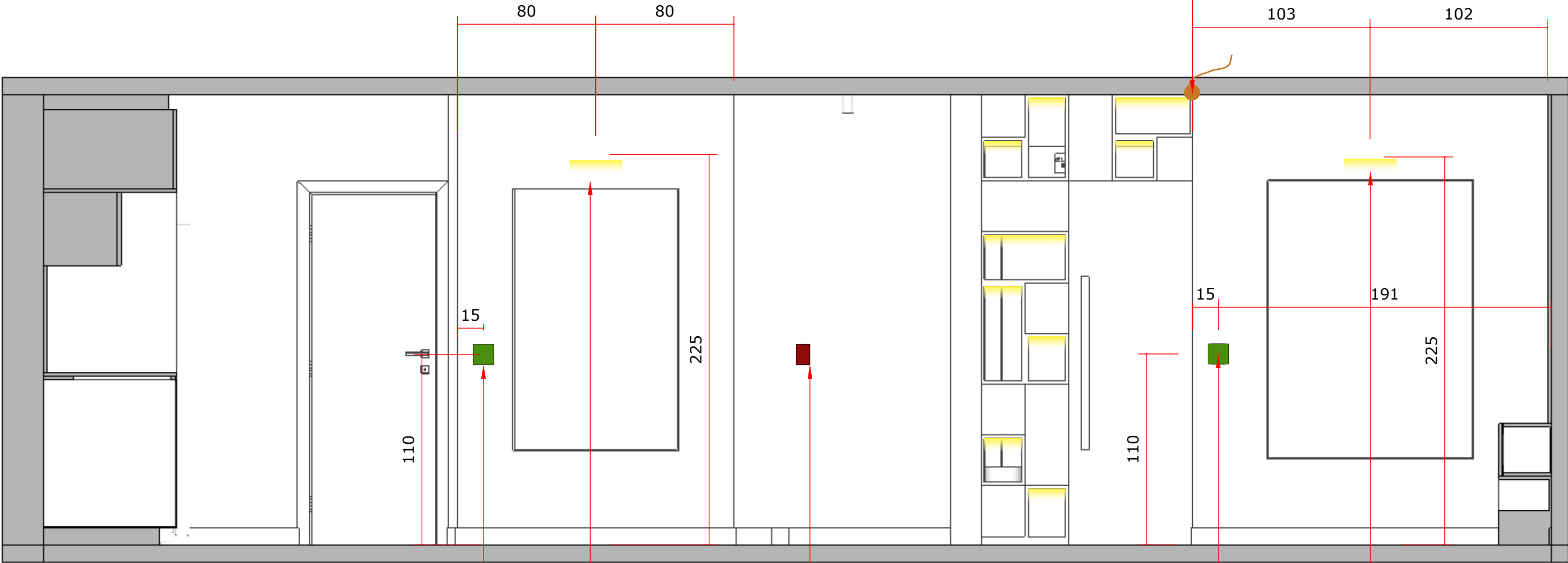
VISTA 4 - PONTOS ELÉTRICOS SALA ESCALA 1:25
