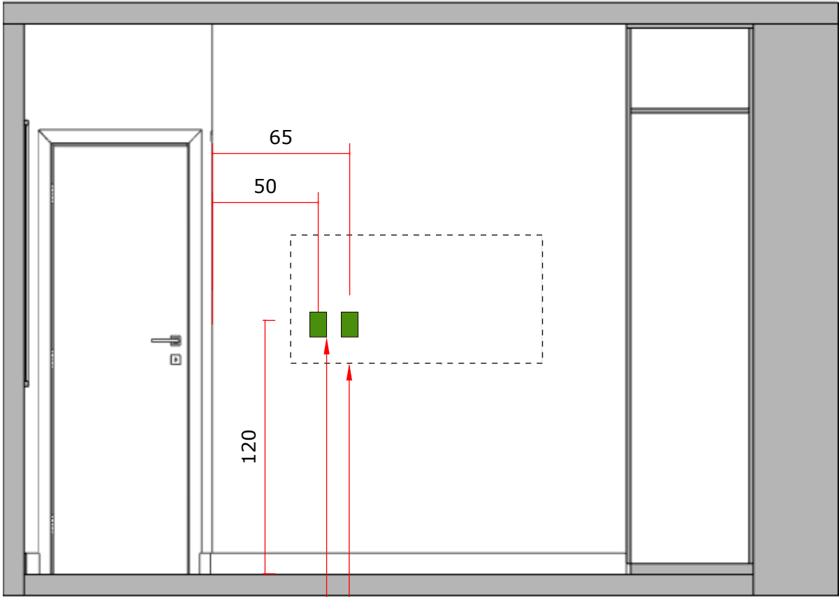
VISTA 3 - PONTOS DE ELÉTRICA SUÍTE 2 ESCALA 1:25
