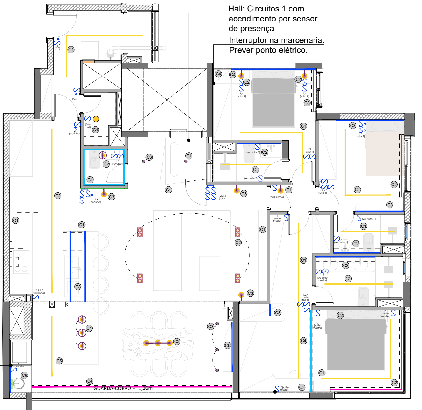
PLANTA DE ILUMINAÇÃO ESCALA 1:75
