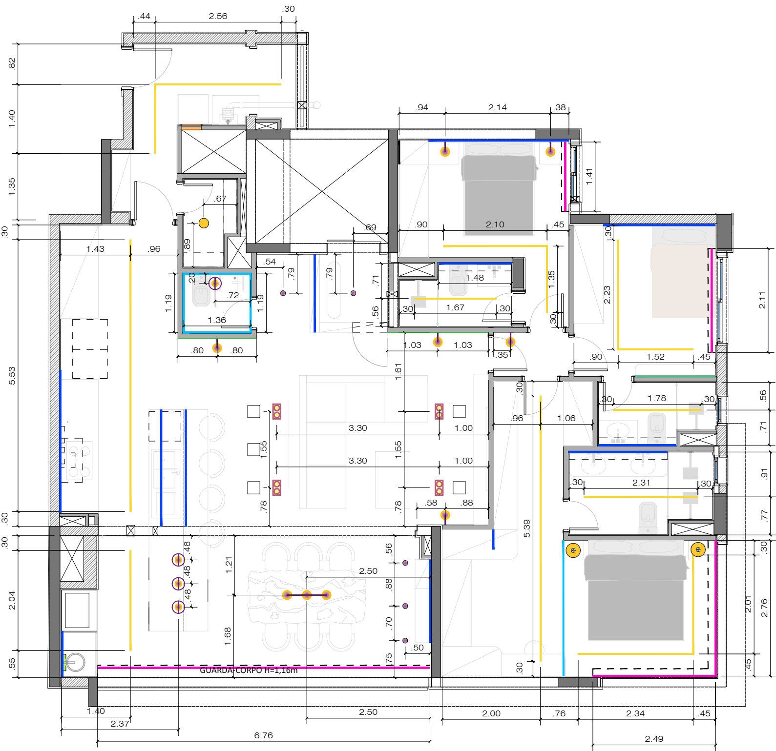
PLANTA DE ILUMINAÇÃO ESCALA 1:75
