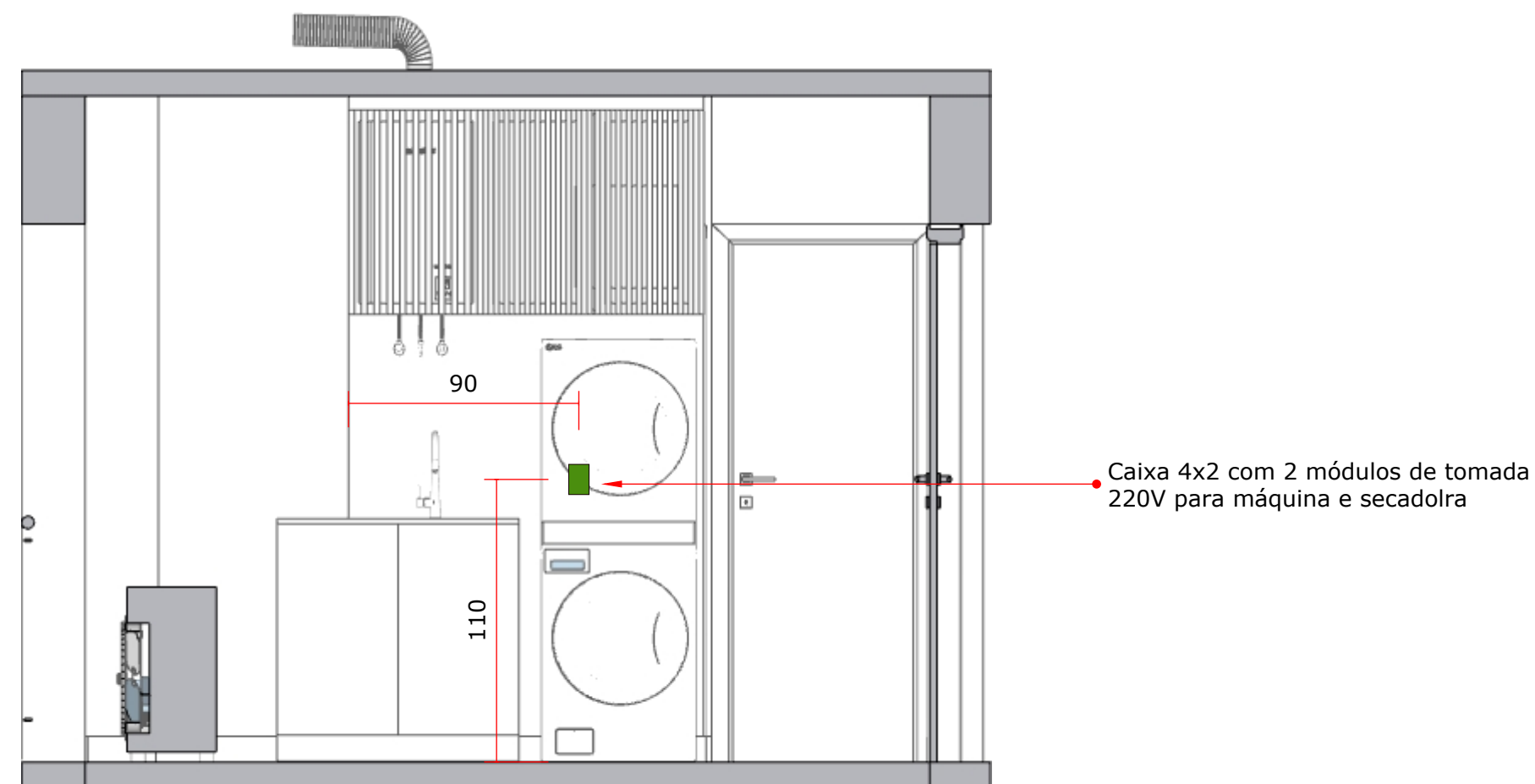
VISTA 1 - PONTOS DE ELÉTRICA LAVANDERIA
