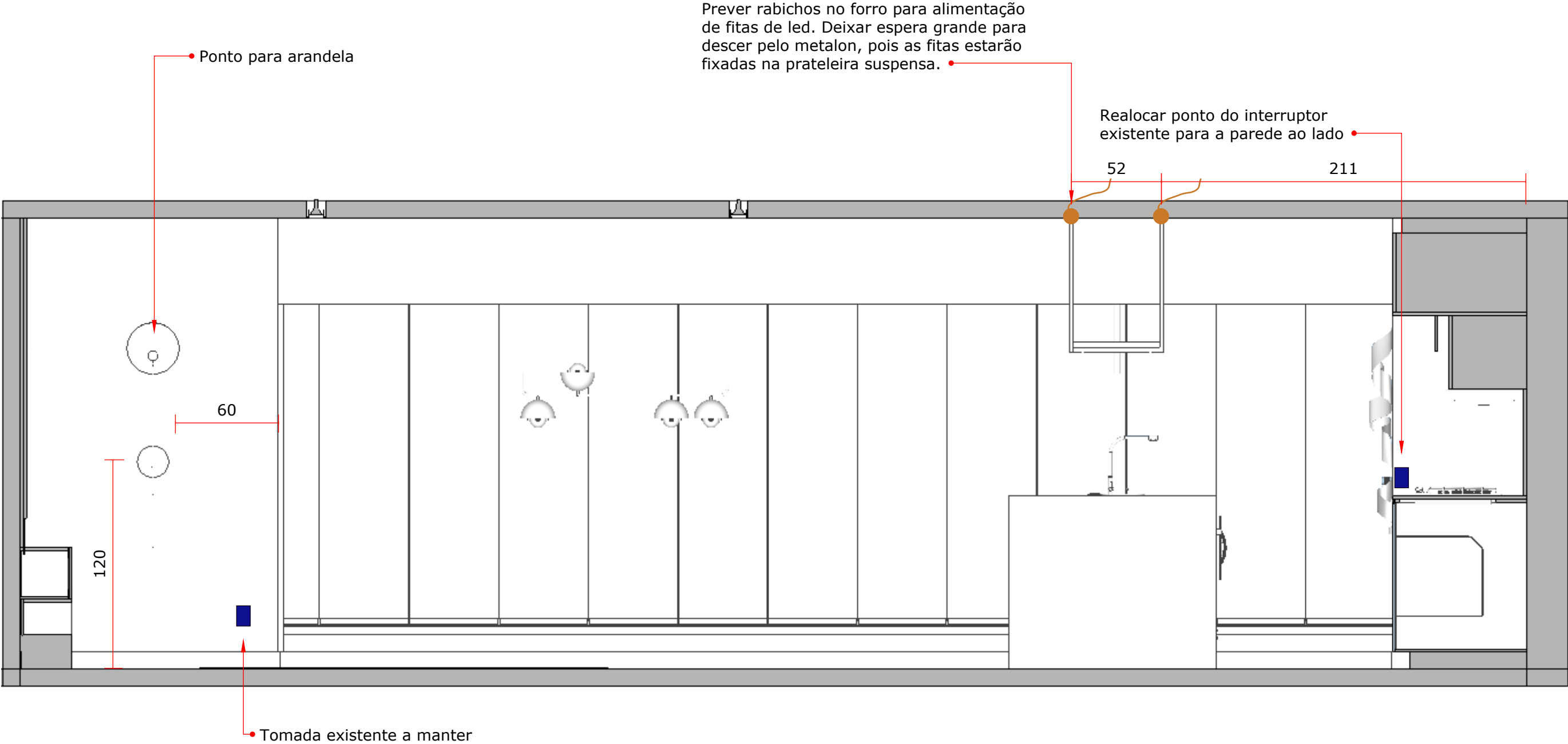
VISTA 2 - PONTOS ELÉTRICOS SALA, VARANDA E COZINHA ESCALA 1:25
