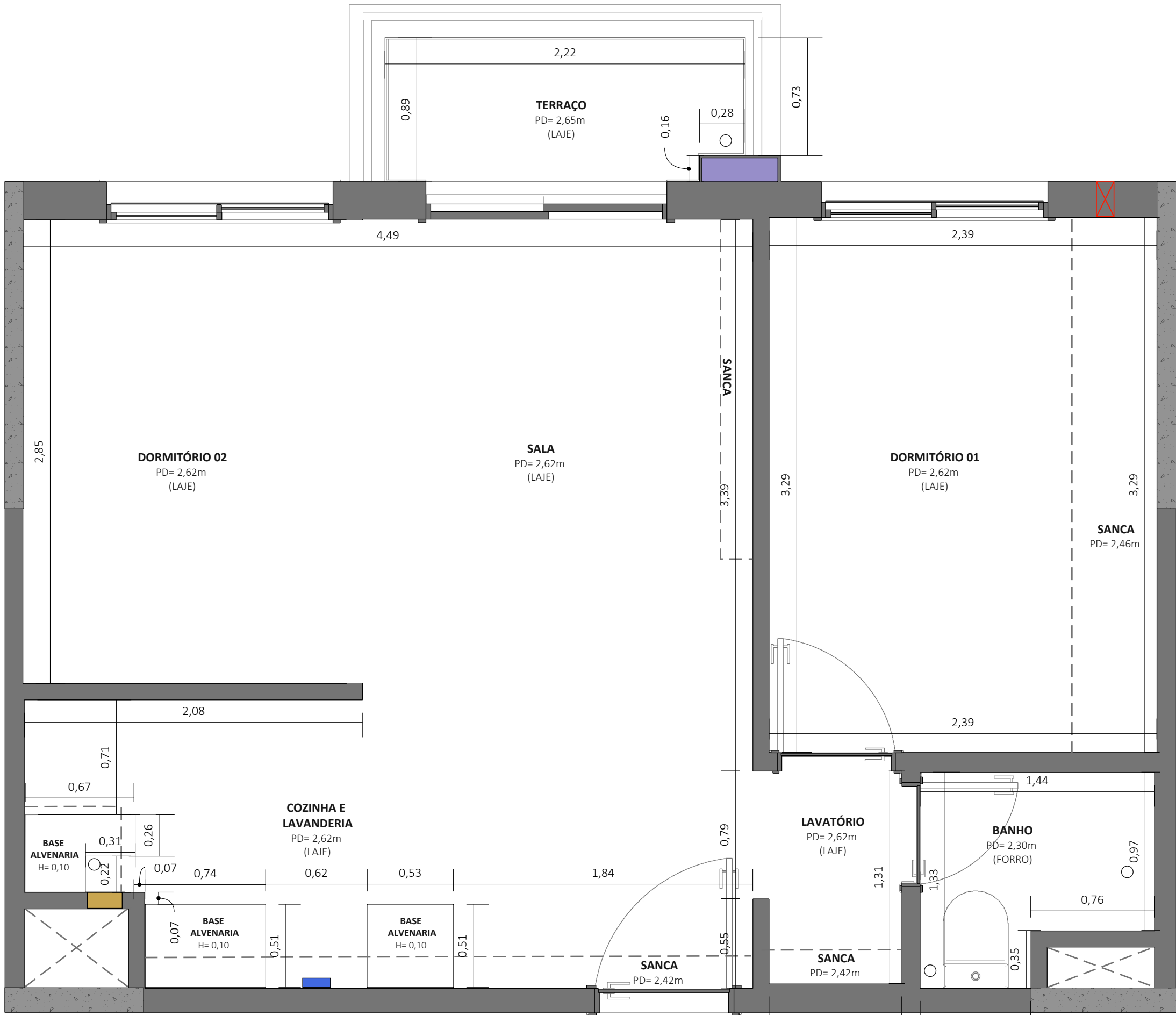
PLANTA ALVENARIA FINAL esc. 1:25 OBS: CONFERIR AS MEDIDAS NO LOCAL
