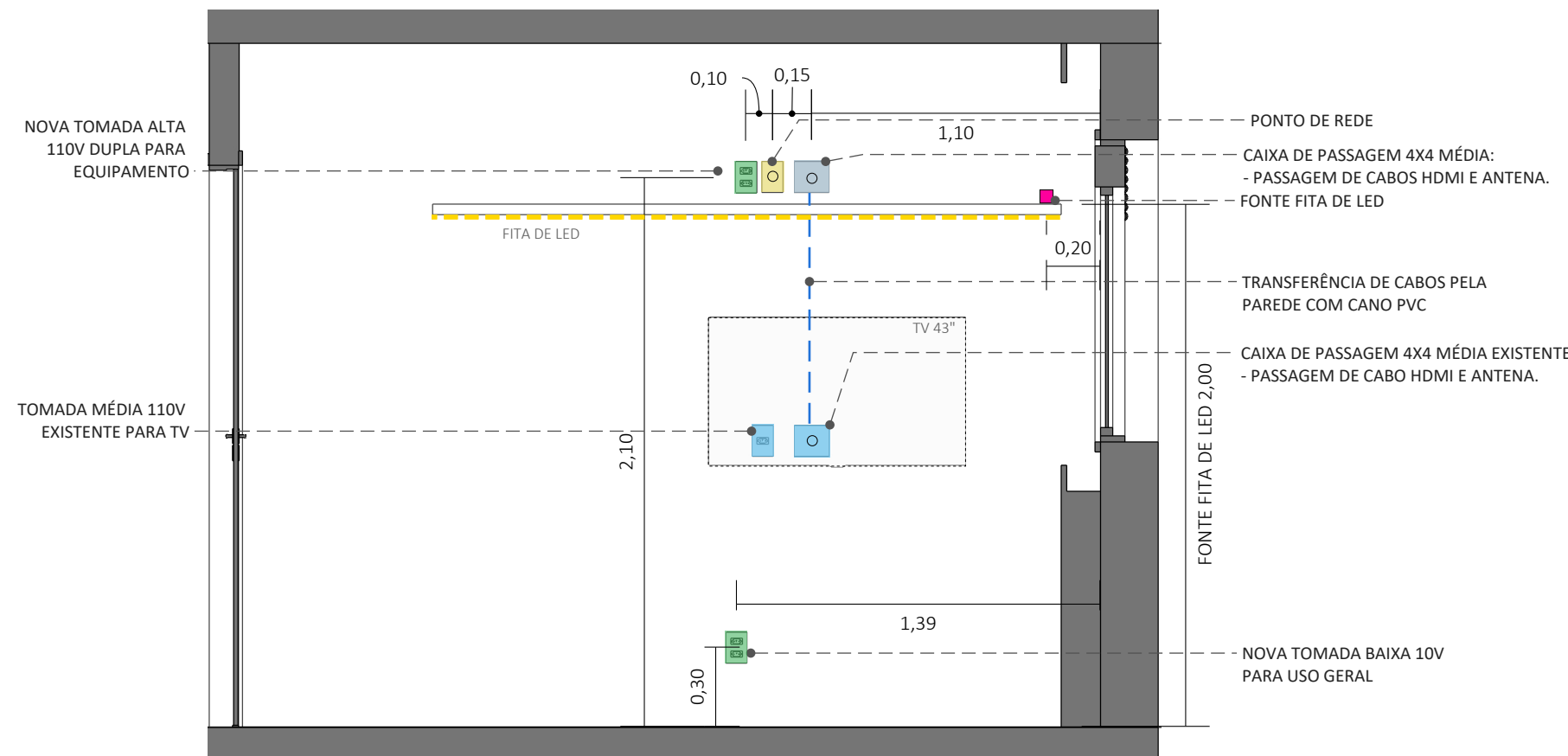
VISTA 08 - ELÉTRICA DORMITÓRIO 01 ESC. 1:25 OBS: CONFERIR AS MEDIDAS NO LOCAL
