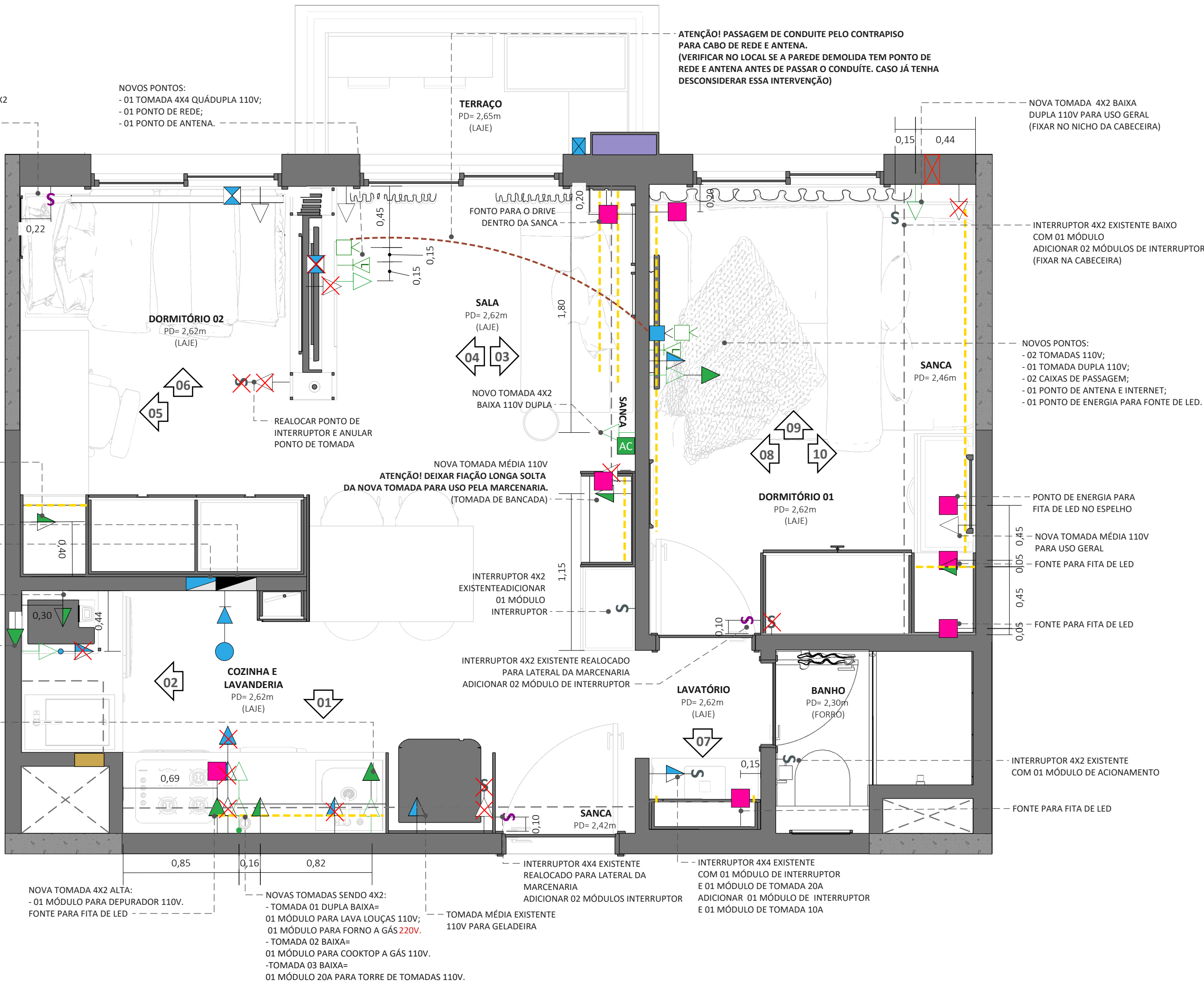
PLANTA ELÉTRICA esc. 1:25 OBS: CONFERIR AS MEDIDAS NO LOCAL
