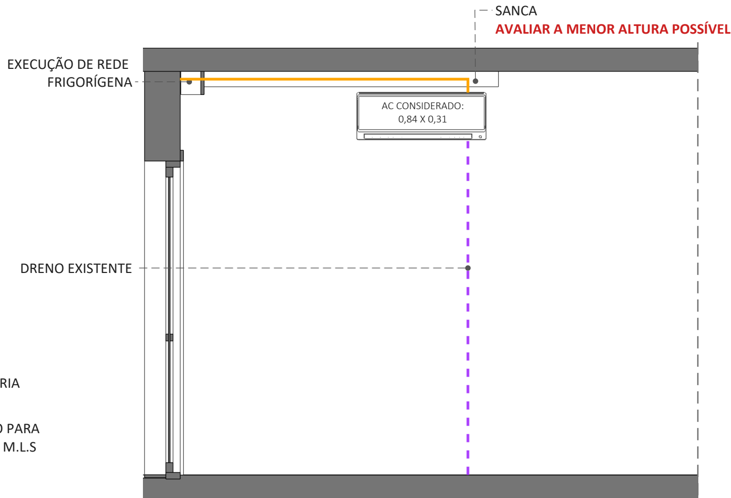
VISTA 03 - AR-CONDICIONADO ESC. 1:25 CONFIRMAR DIMENSÕES DE ACORDO COM EQUIPAMENTOS DE AR-CONDICIONADO COMPRADOS
