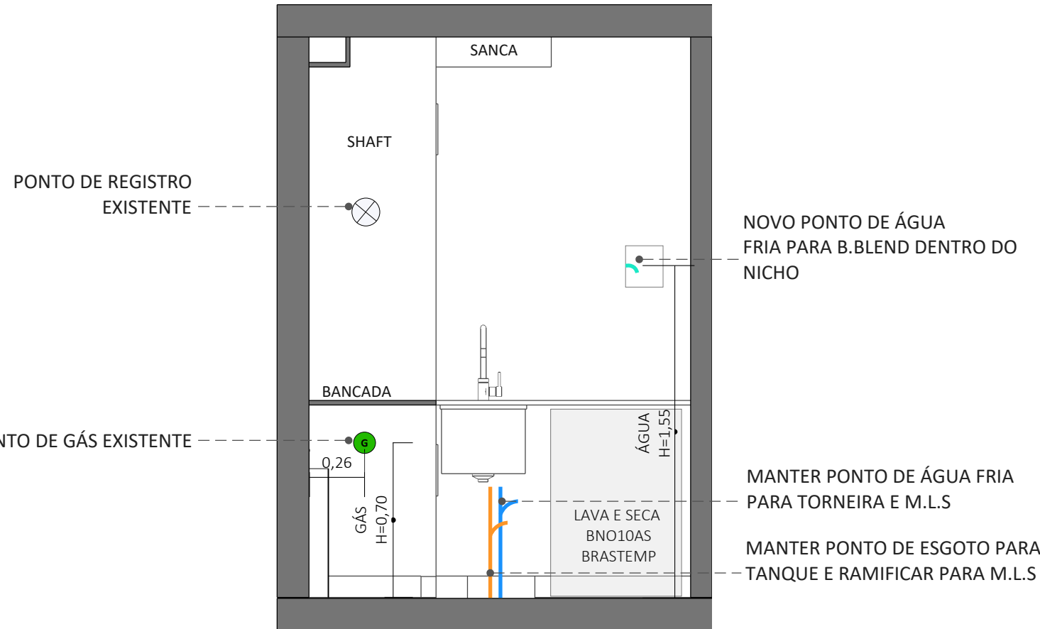
VISTA 01 - HIDRÁULICA DA LAVANDERIA ESC. 1:25
