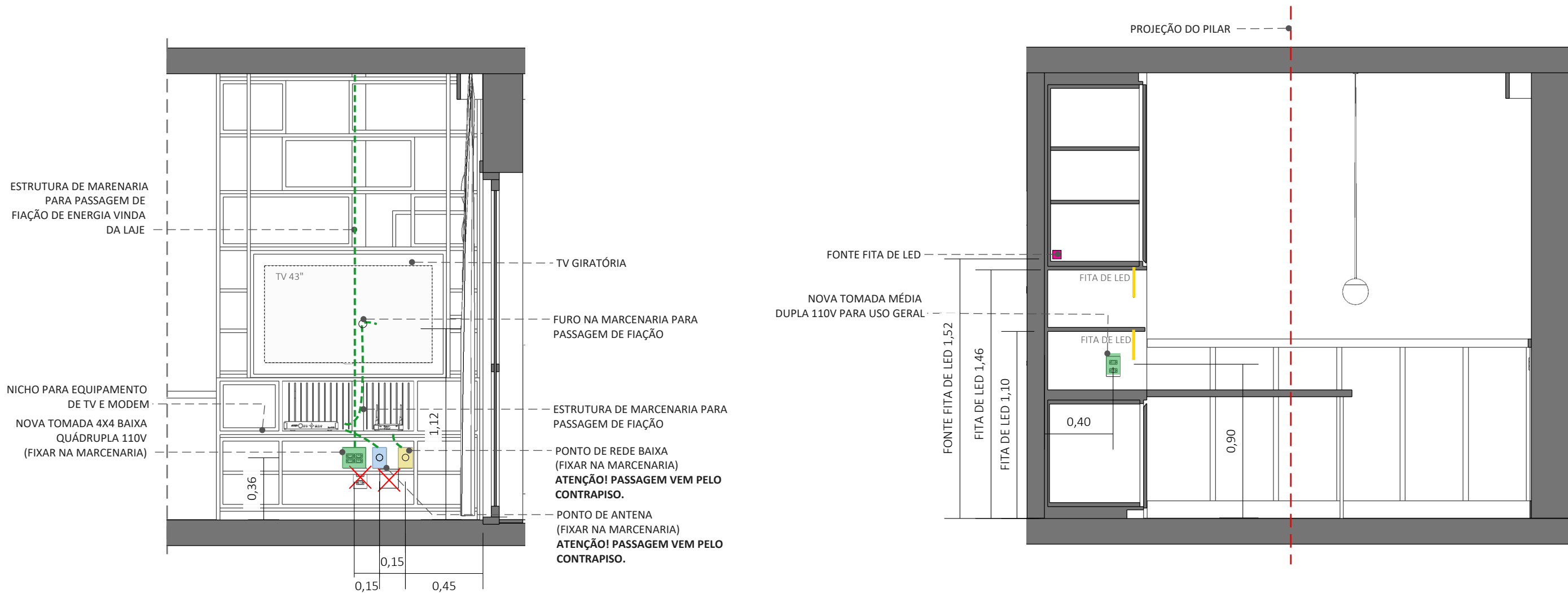
VISTA 04 - ELÉTRICA SALA ESC. 1:25 OBS: CONFERIR AS MEDIDAS NO LOCAL
