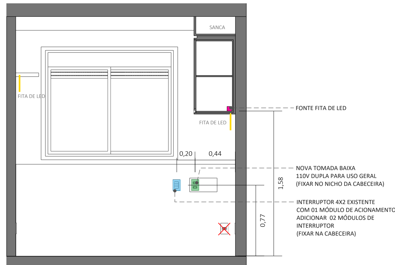
VISTA 09 - ELÉTRICA DORMITÓRIO 01 ESC. 1:25 OBS: CONFERIR AS MEDIDAS NO LOCAL
