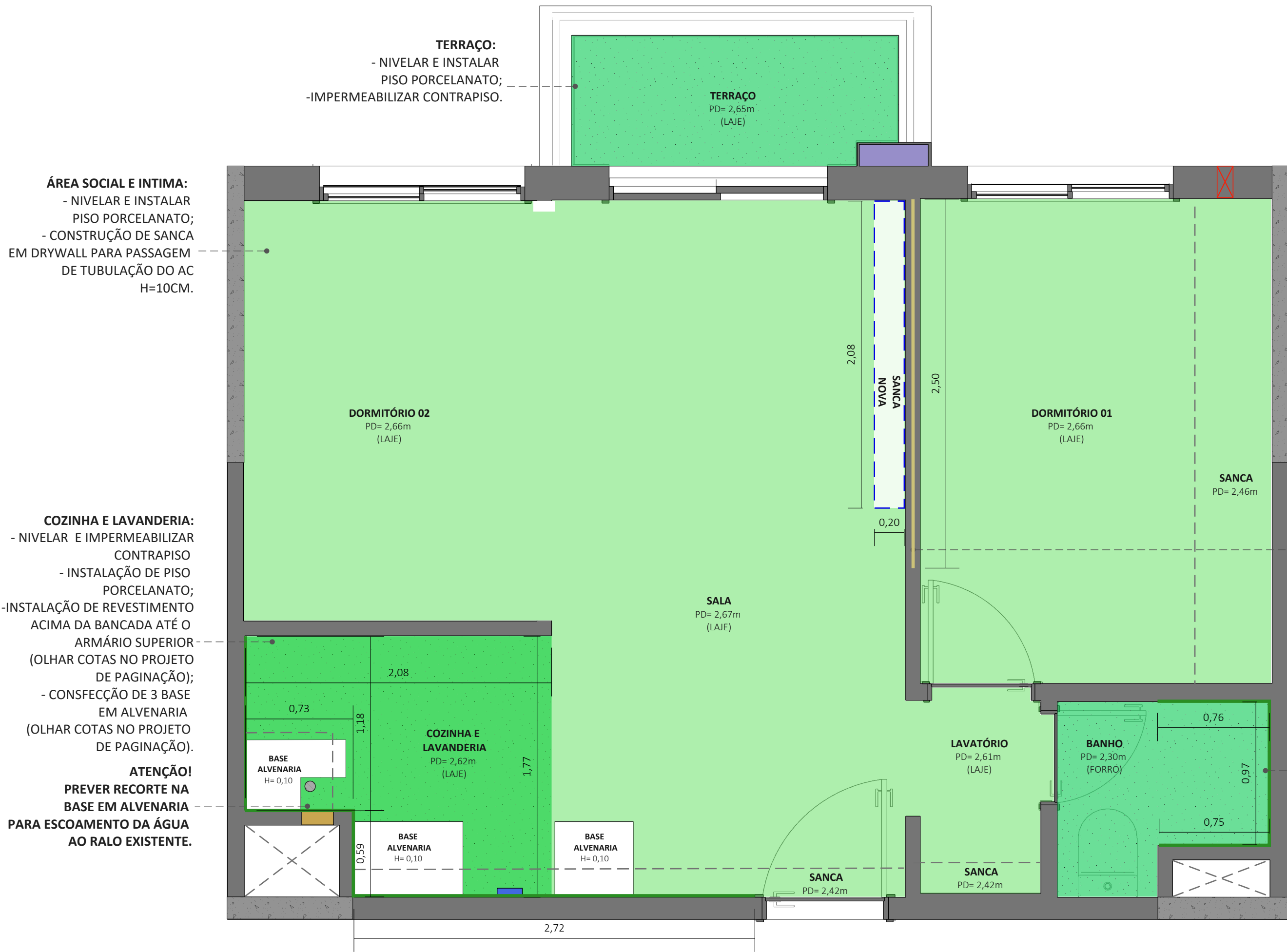
PLANTA CONSTRUIR esc. 1:25 OBS: CONFERIR AS MEDIDAS NO LOCAL
