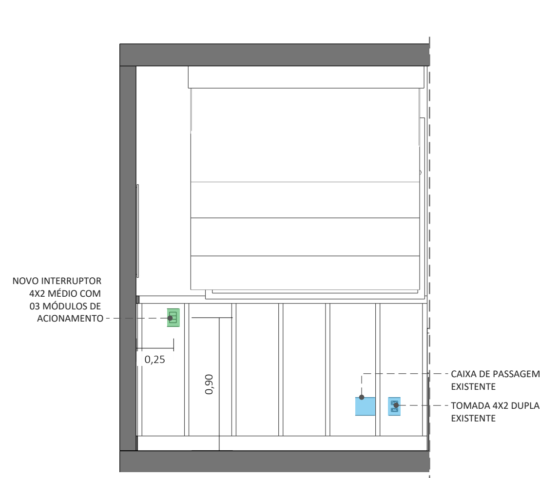
VISTA 06 - ELÉTRICA DORMITÓRIO 02 ESC. 1:25 OBS: CONFERIR AS MEDIDAS NO LOCAL
