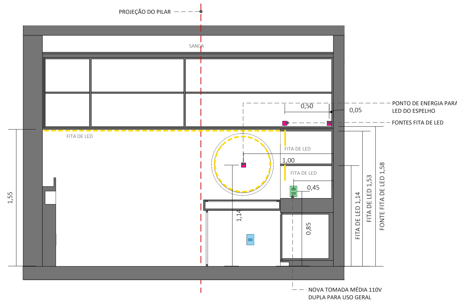
VISTA 10 - ELÉTRICA DORMITÓRIO 01 ESC. 1:25 OBS: CONFERIR AS MEDIDAS NO LOCAL
