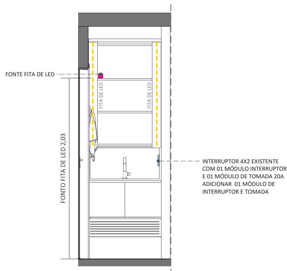
VISTA 07 - ELÉTRICA LAVATÓRIO ESC. 1:25 OBS: CONFERIR AS MEDIDAS NO LOCAL
