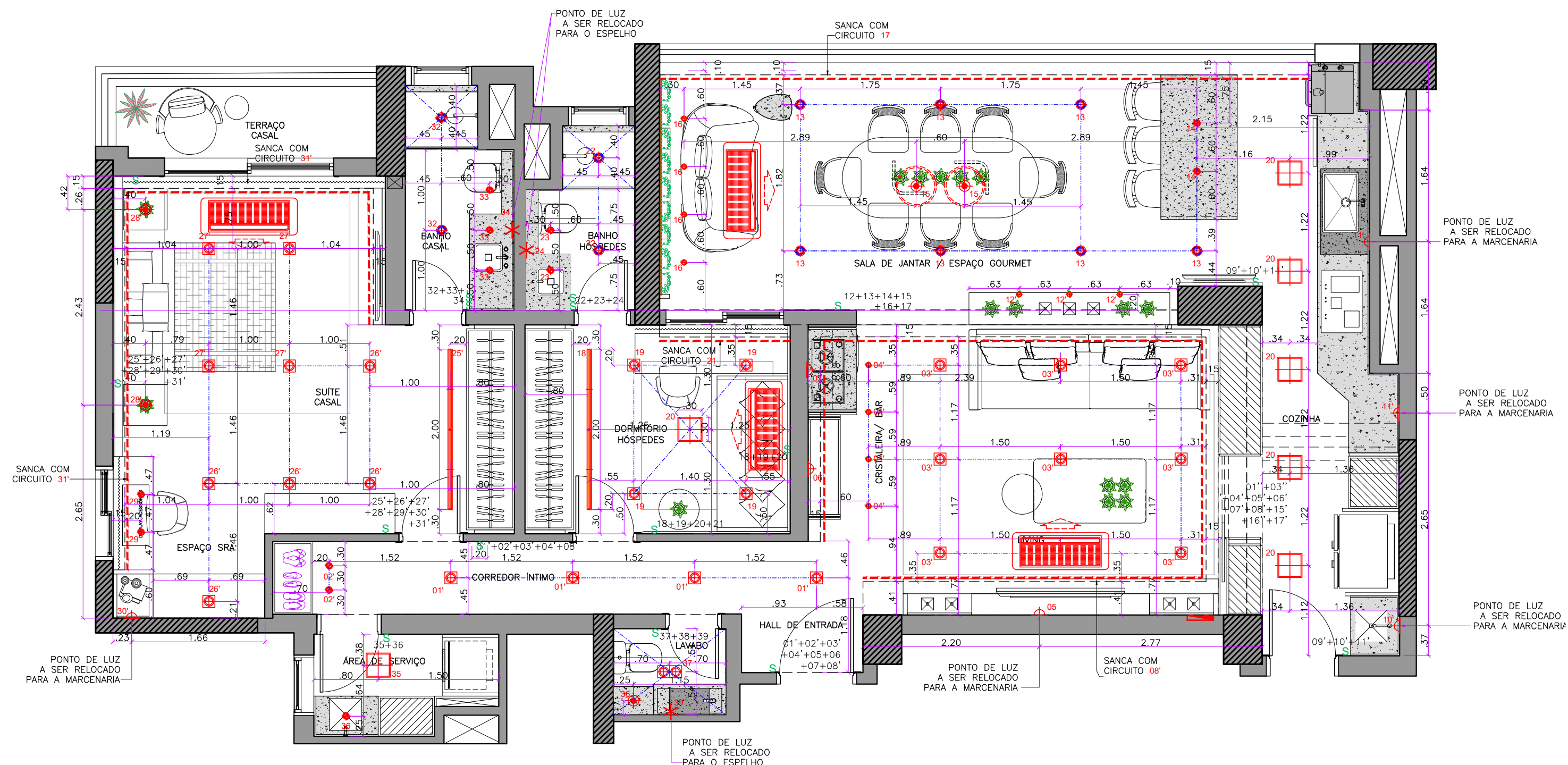
PLANTA DE ILUMINAÇÃO esc 1:50
