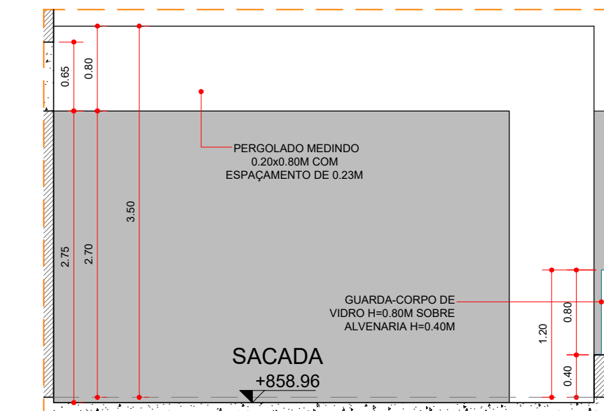
DETALHE PERGOLADO SACADA SUÍTE CASAL ESCALA 1:50
