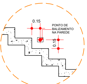
DETALHE ILUMINAÇÃO NA ESCADA ESCALA 1:25
