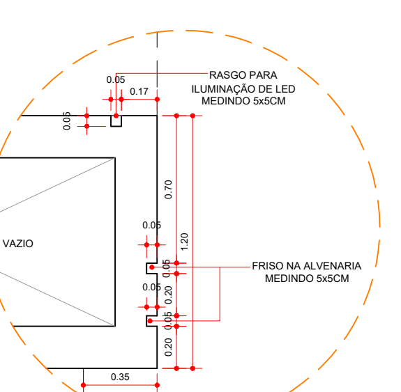
DETALHE FRISOS NA FACHADA ESCALA 1:25
