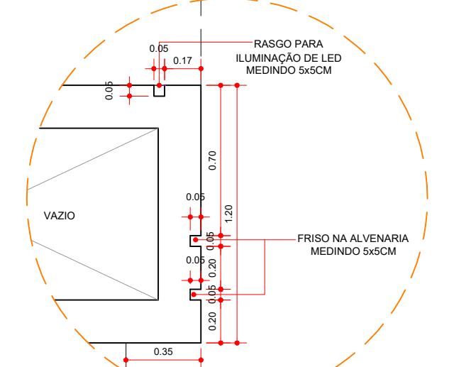
DETALHE FRISOS NA FACHADA ESCALA 1:25
