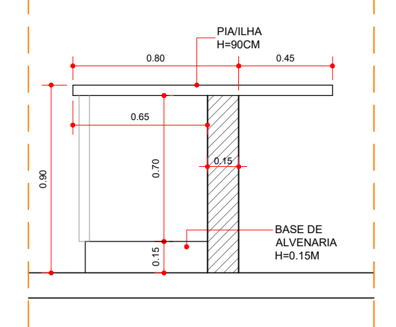
DETALHE DA PIA COZINHA ESCALA 1:25
