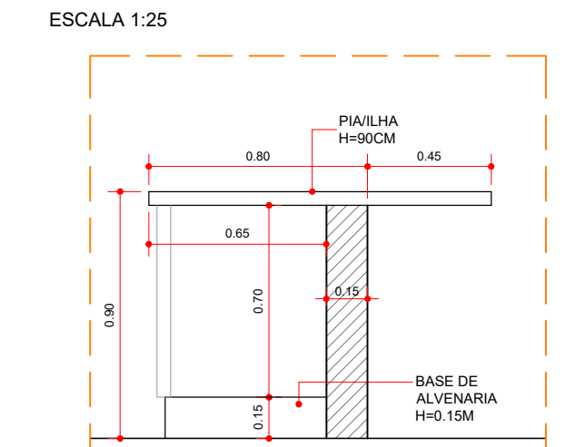
DETALHE DA PIA COZINHA ESCALA 1:25
