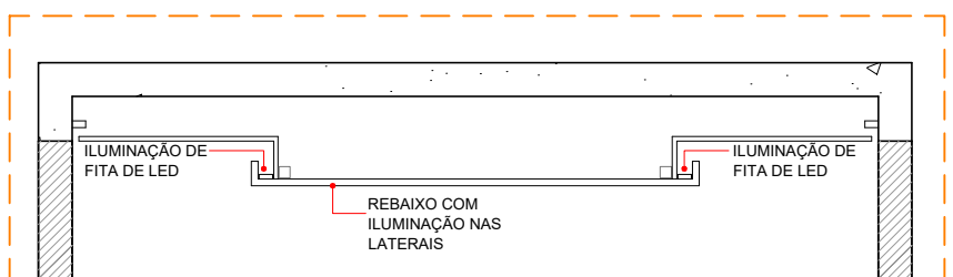
DETALHE DO REBAIXO COM ILUMINAÇÃO DE FITA DE LED ESCALA 1:25
