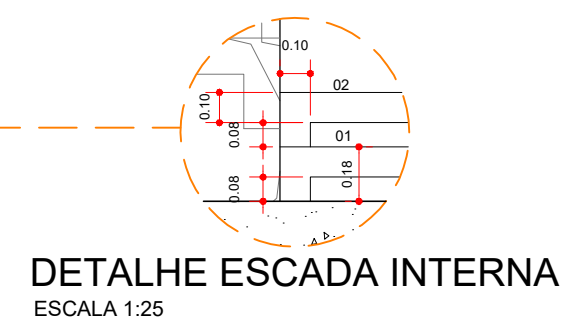
DETALHE ESCADA INTERNA ESCALA 1:25
