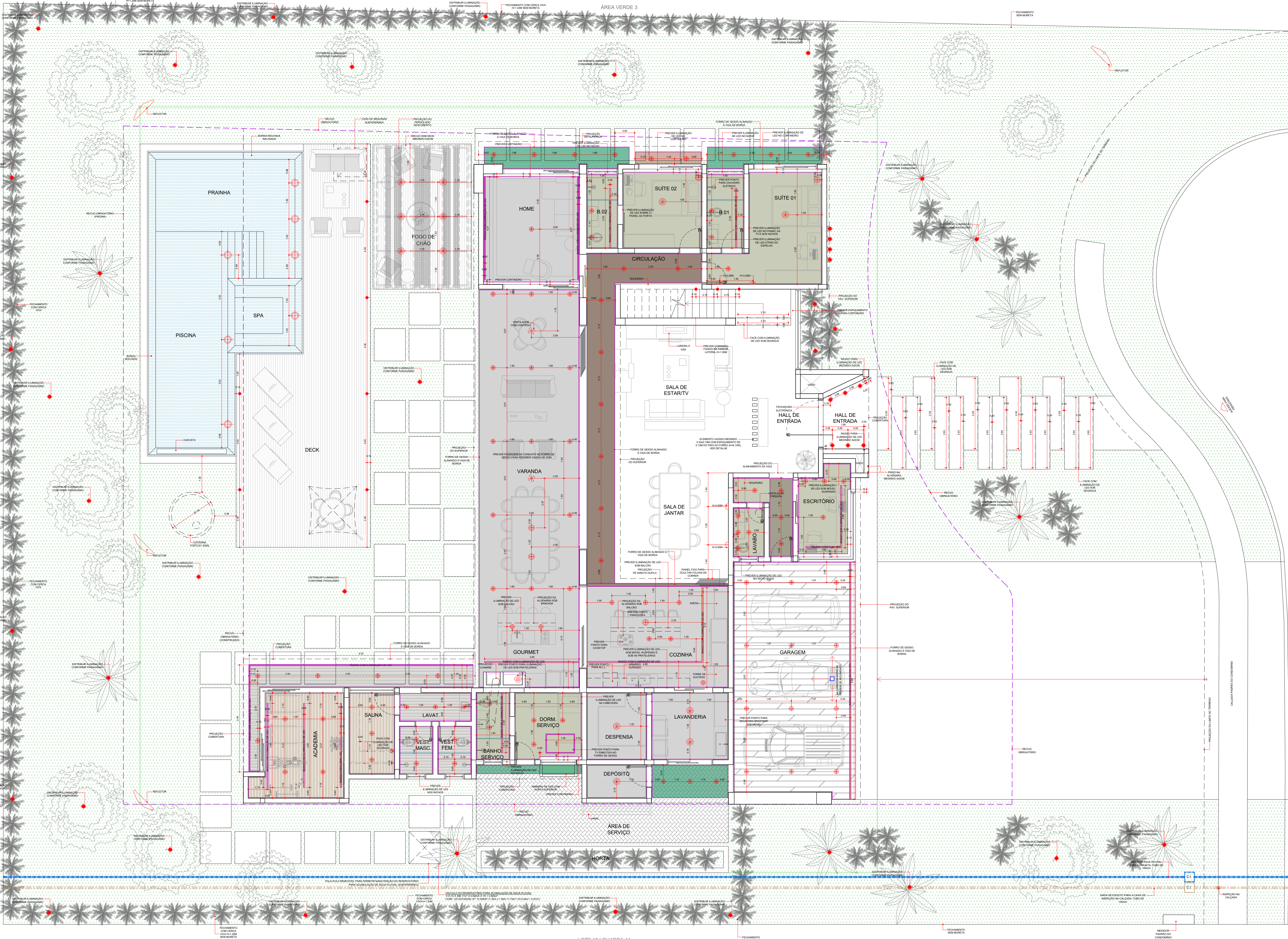
PLANTA (pav. térreo)
