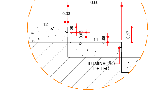
DETALHE ESCADA FACHADA ESCALA 1:25
