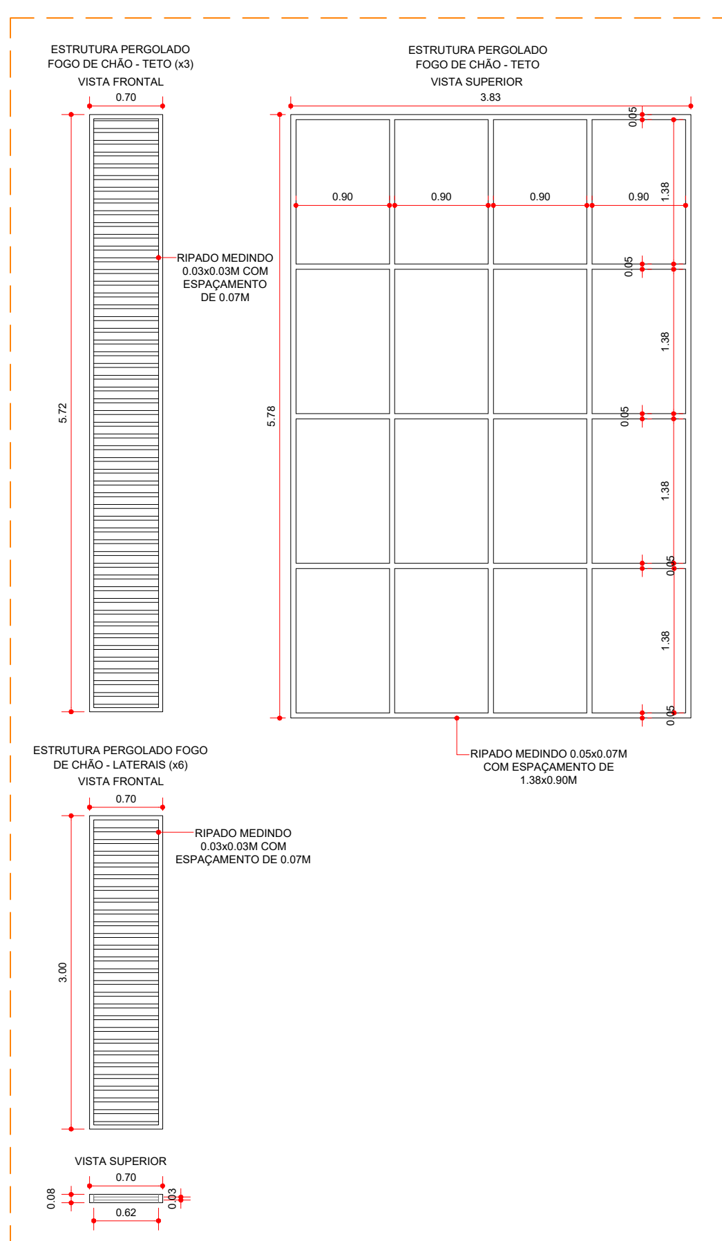
DETALHE PERGOLADO DO FOGO DE CHÃO ESCALA 1:50
