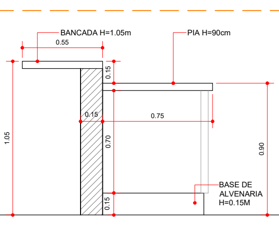
DET. PIA/BANCADA GOURMET ESCALA 1:25
