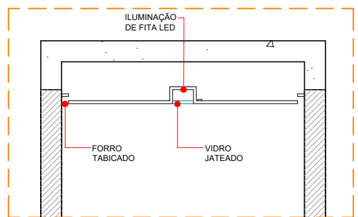
DETALHE RASGO COM ILUMINAÇÃO DE LED E VIDRO JATEADO OU CANALETA DE LED EMBUTIDA NO FORRO DE GESSO ESCALA 1:25
