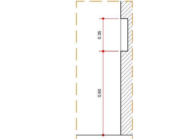
DETALHE NICHOS TODOS OS BANHEIROS ESCALA 1:25
