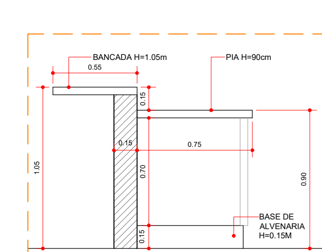
DET. PIA/BANCADA GOURMET ESCALA 1:25
