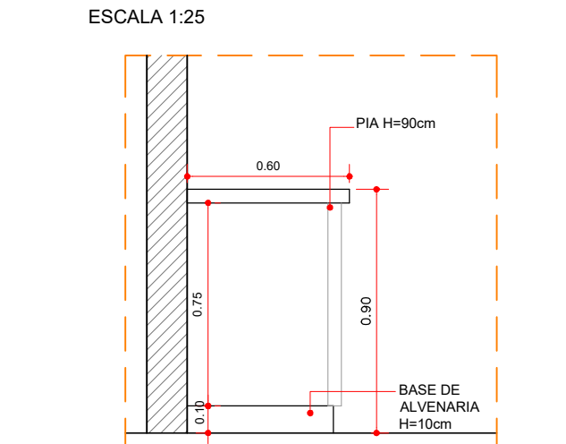
DETALHE DA PIA ESCALA 1:25
