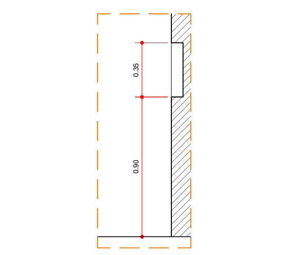
DETALHE NICHOS TODOS OS BANHEIROS ESCALA 1:25
