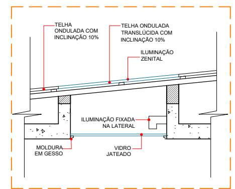
DETALHE DA ILUMINAÇÃO ZENITAL ESCALA 1:25
