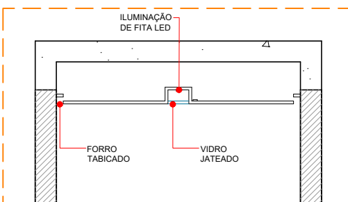
HE RASGO COM ILUMINAÇÃO DE LED E VIDRO JATEADO OU ETA DE LED EMBUTIDA NO FORRO DE GESSO
