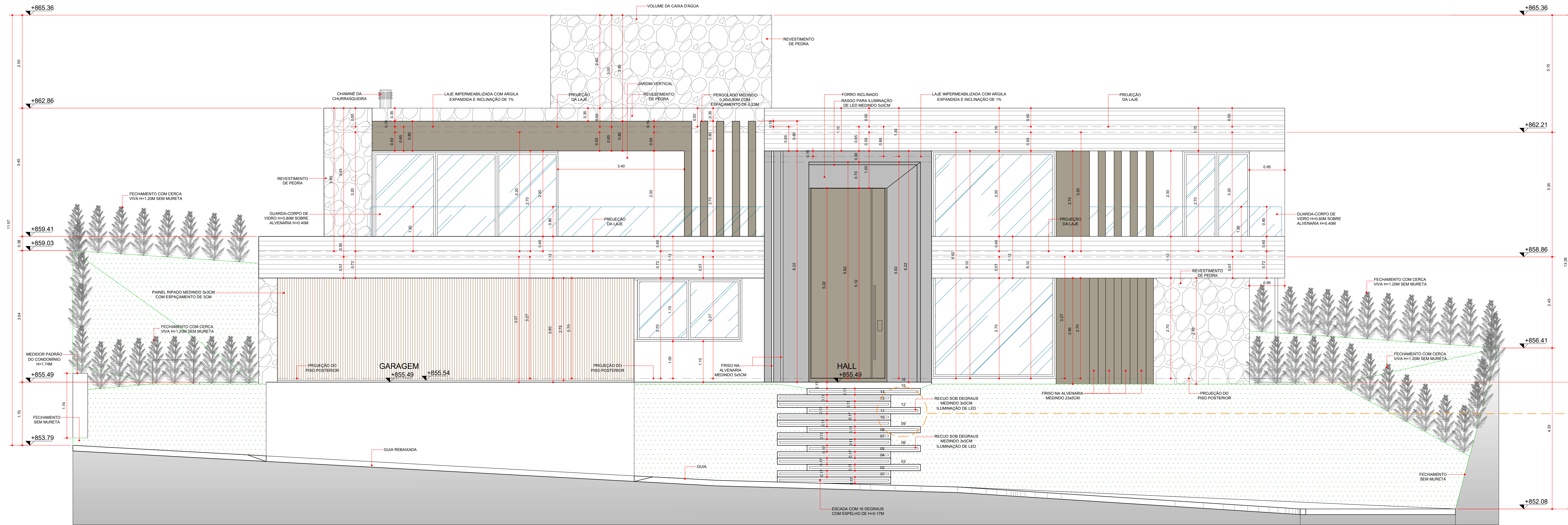
FACHADA ESC. 1:50
