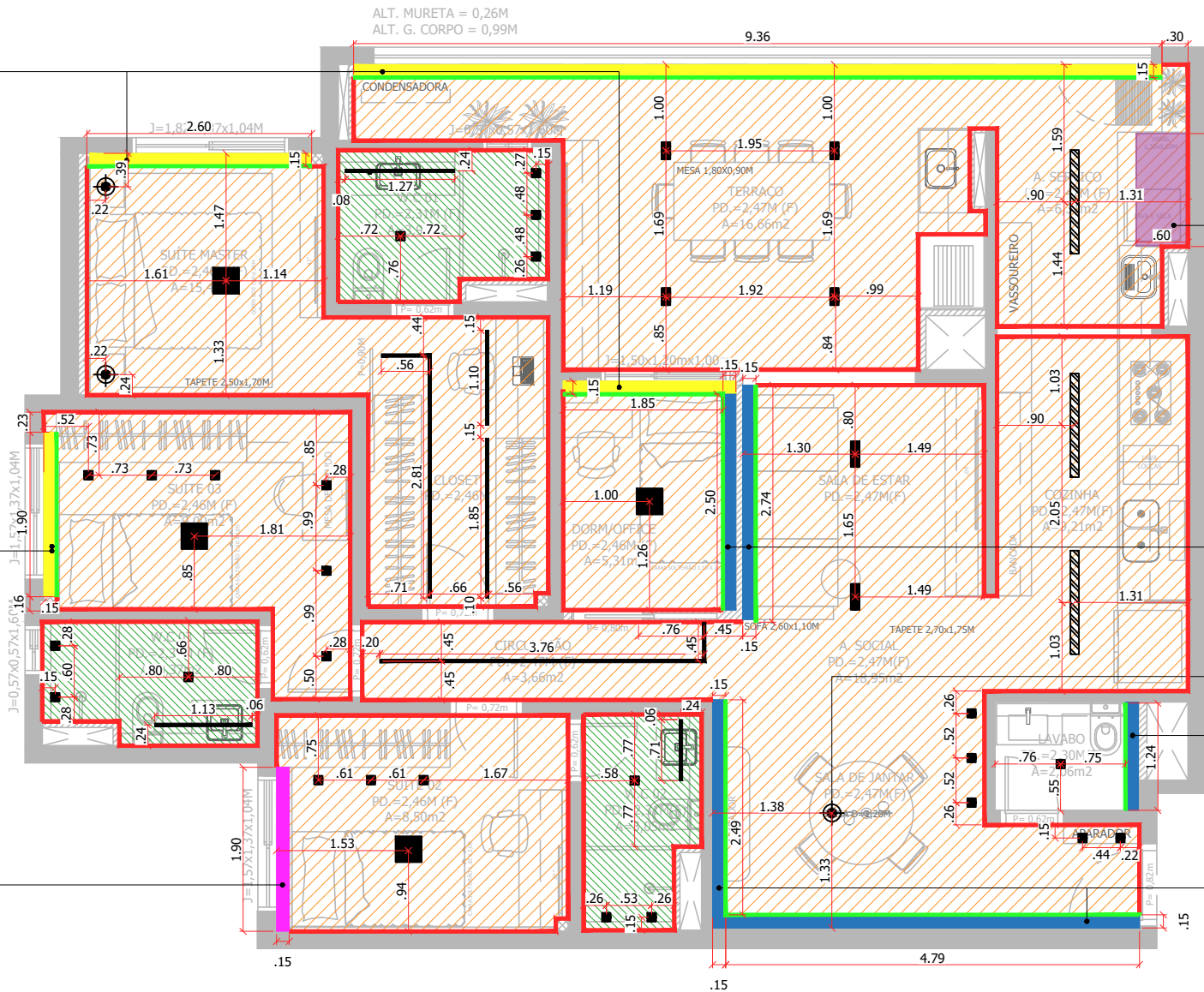
PLANTA BAIXA - FORRO ESC.: 1:75 ÁREA.:114,00m2
