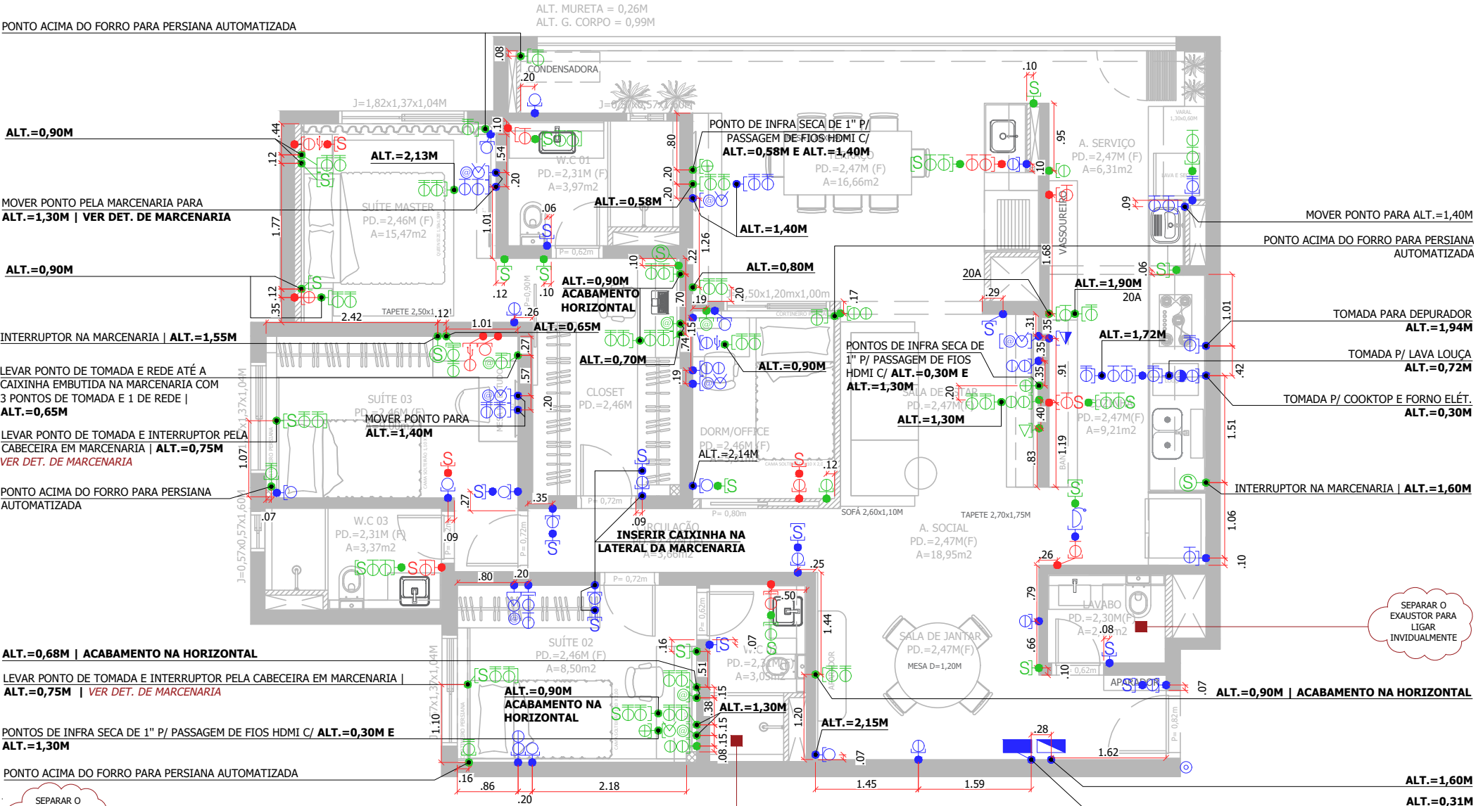
PLANTA BAIXA - PONTOS ELÉTRICOS ESC.: 1:75 ÁREA.:114,00m2
