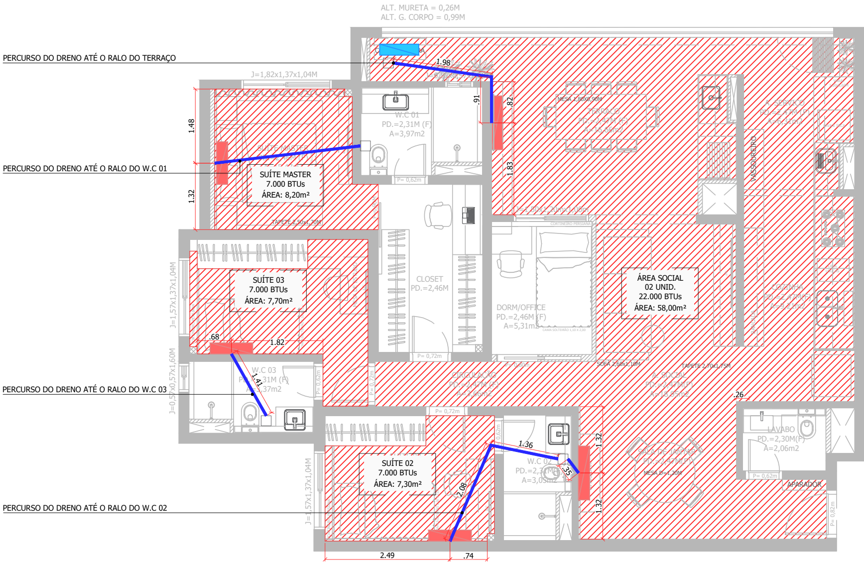
PLANTA BAIXA - AR CONDICIONADO ESC.: 1:75 ÁREA.:114,00m2
