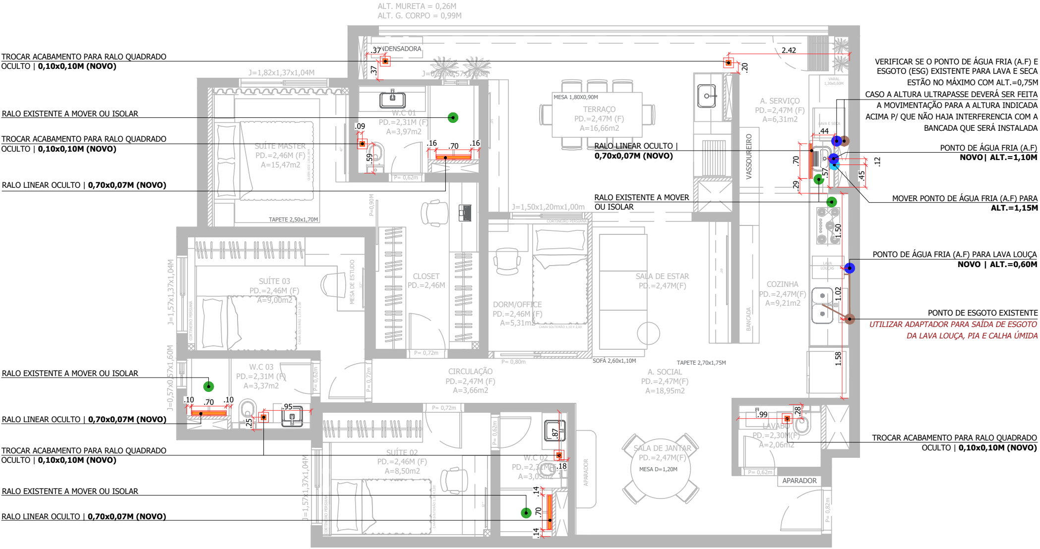
PLANTA BAIXA - PONTOS HIDRÁULICOS ESC.: 1:75 ÁREA.:114,00m2
