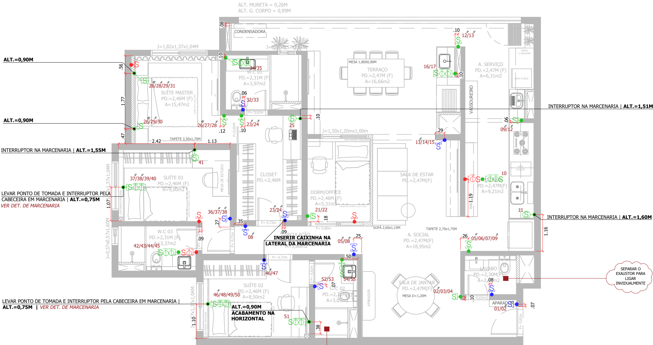
PLANTA BAIXA - INTERRUPTORES ESC.: 1:75 ÁREA.:114,00m2
