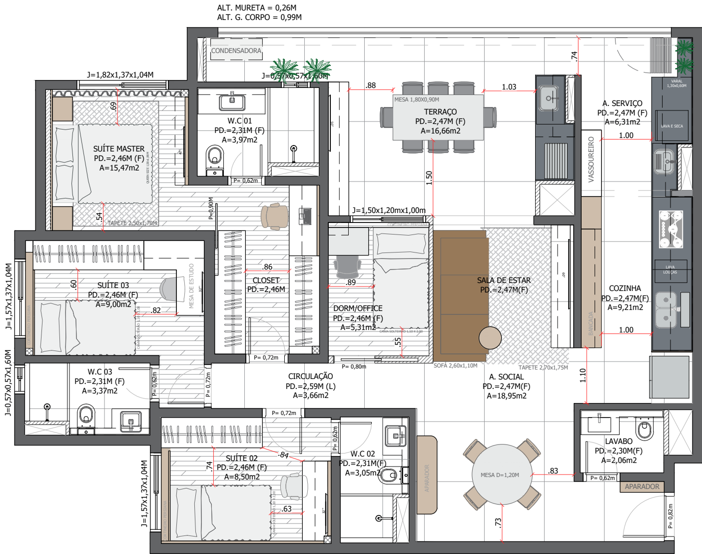
PLANTA BAIXA - LAYOUT ESC.: 1:75 ÁREA.:114,00m2
