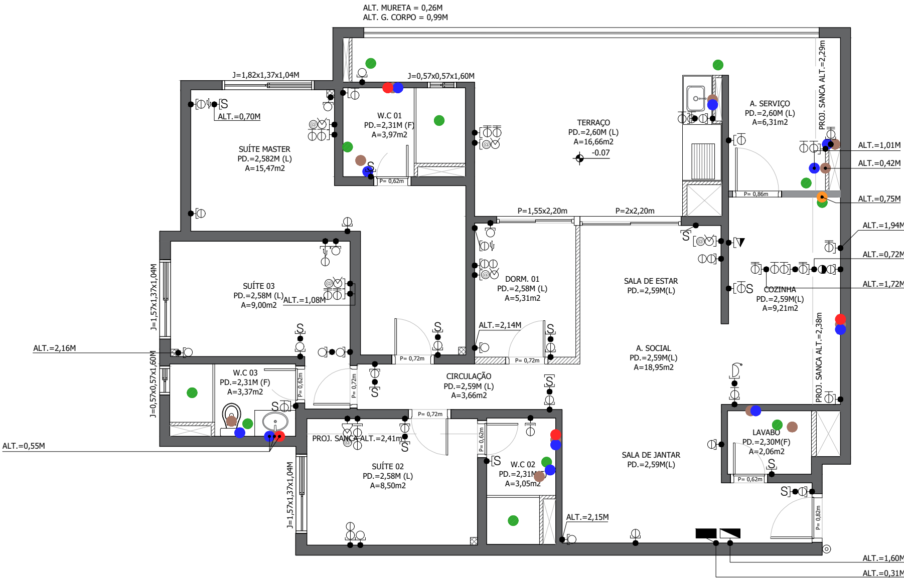
PLANTA BAIXA - LEVANTAMENTO TÉCNICO ESC.: 1:75 ÁREA.:114,00m2
