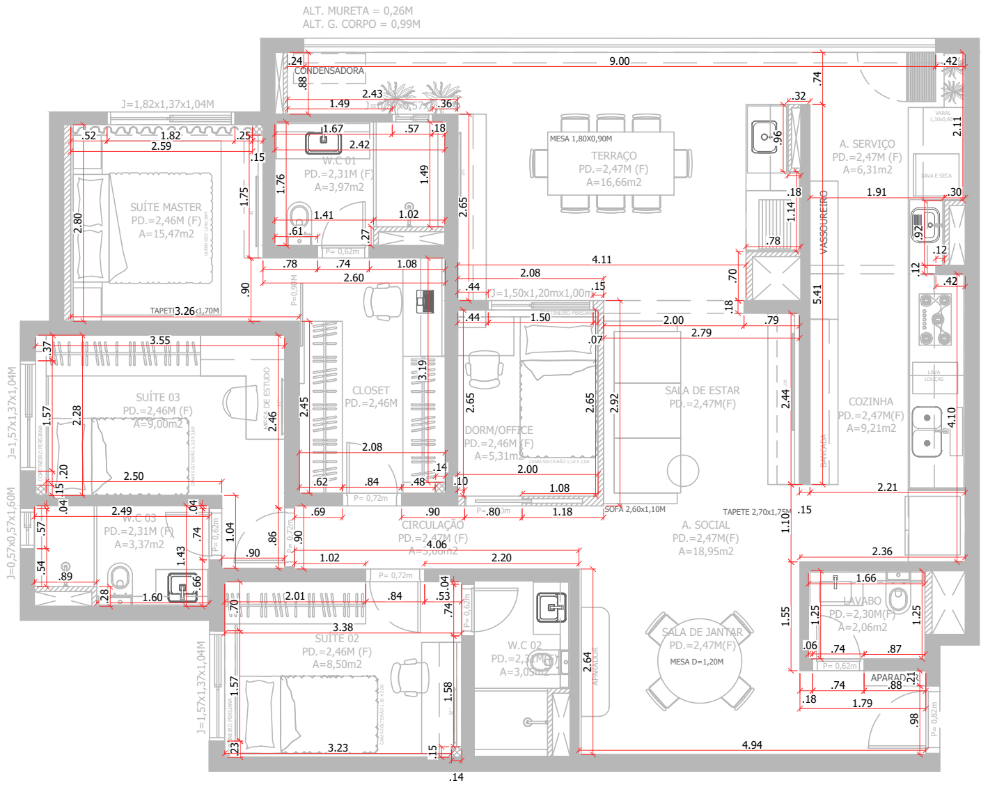
PLANTA BAIXA - ARQUITETURA ESCALA: 1:75 ÁREA: 114,00m2
