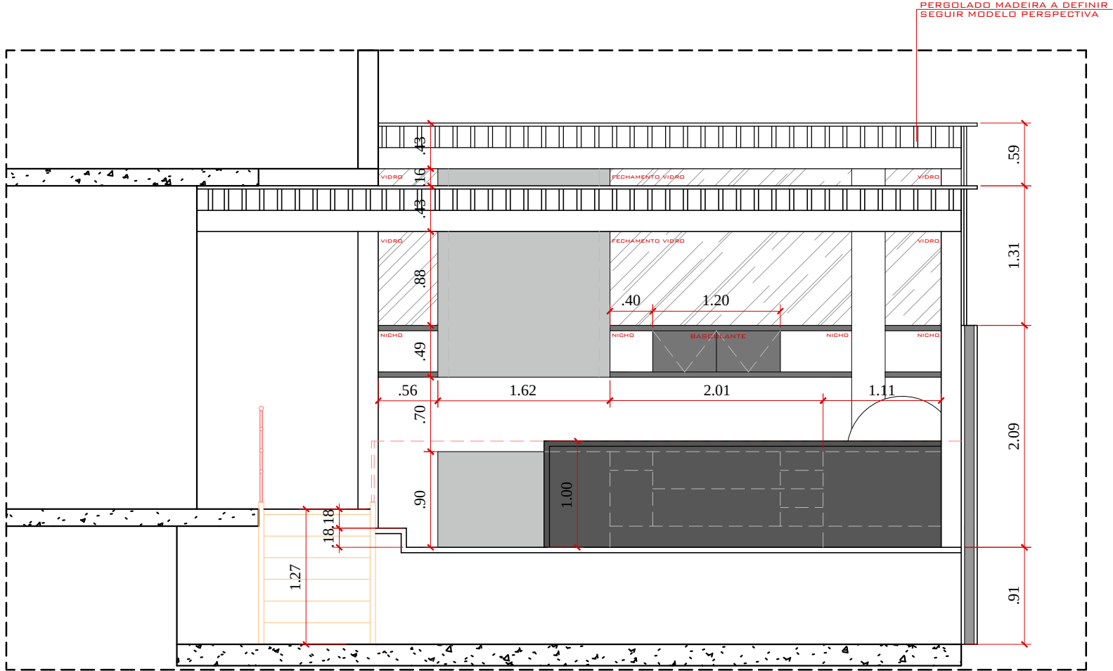
ELEVAÇÃO D
