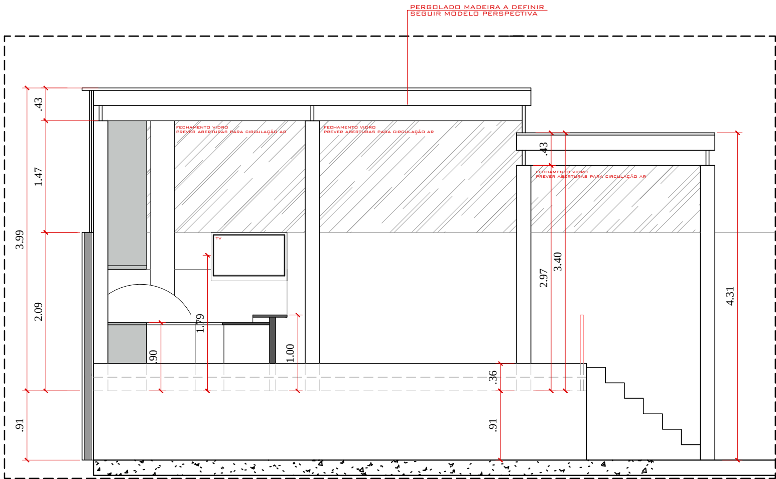
ELEVAÇÃO C
