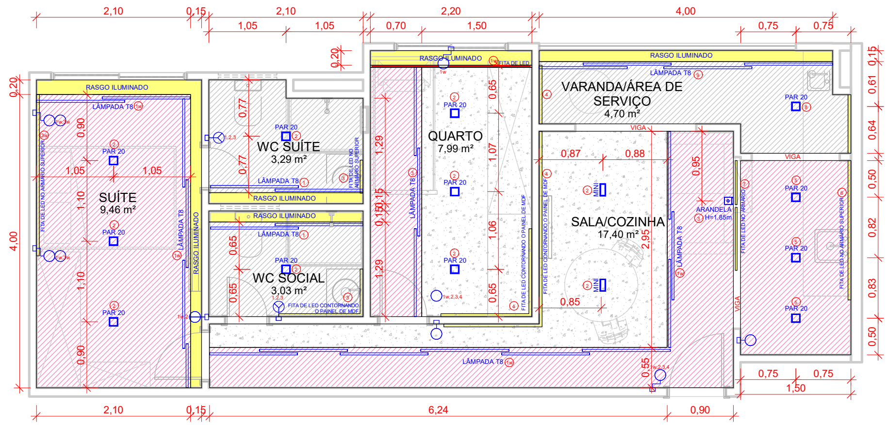
1 PLANTA BAIXA ESCALA 1 : 50
