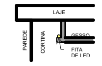
3 DET. CORTINEIRO QUARTO ESCALA 1 : 25
