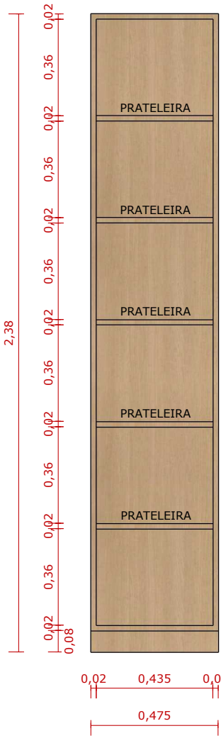
VISTA INTERNA ESC. 1:20
