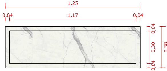
VISTA SUPERIOR ESC. 1:20
