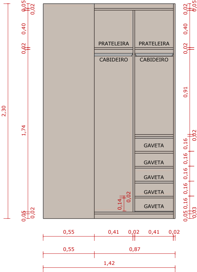
VISTA FRONTAL INTERNA ESC. 1:25
