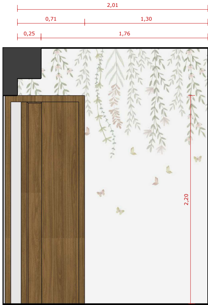
VISTA A ESC. 1:25
