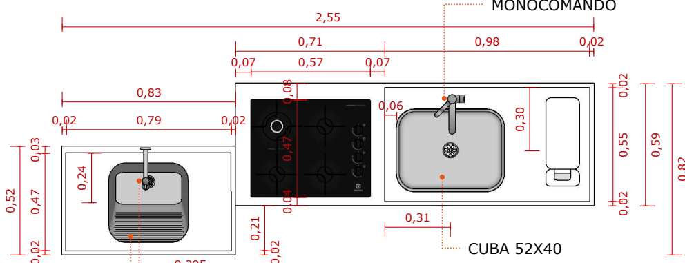
VISTA SUPERIOR ESC. 1:25
