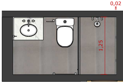
PLANTA BANHO ESC. 1:50
