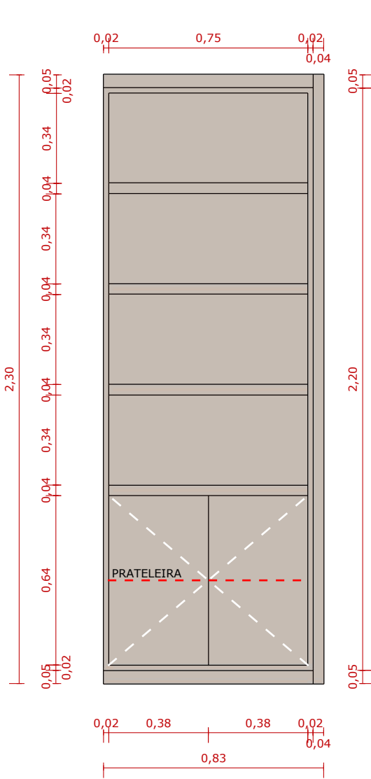
VISTA FRONTAL ESC. 1:20
