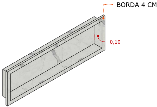
PERSPECTIVA SEM ESCALA
