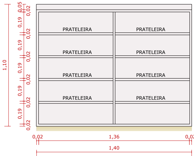
VISTA INTERNA ESC. 1:20
