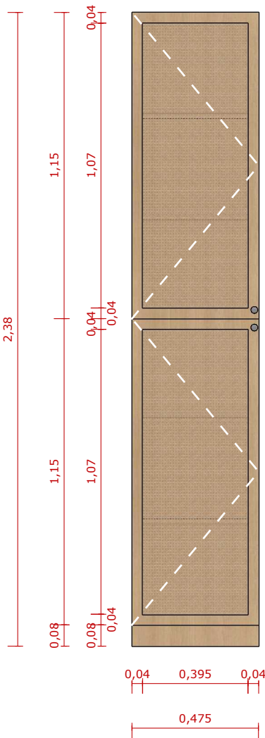
VISTA FRONTAL ESC. 1:20
