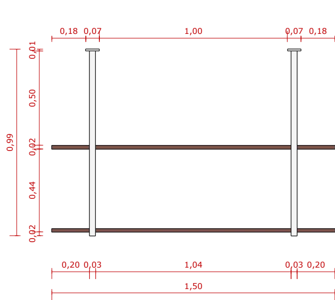
VISTA FRONTAL ESC. 1:20
