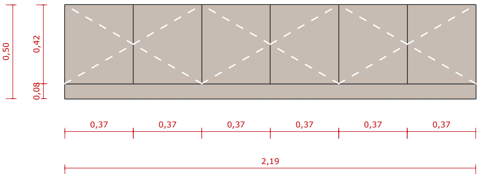
VISTA FRONTAL ESC. 1:20
