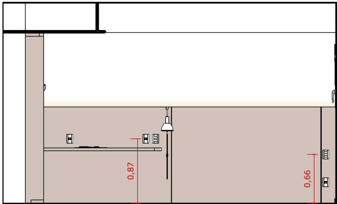
VISTA D ESC. 1:50
