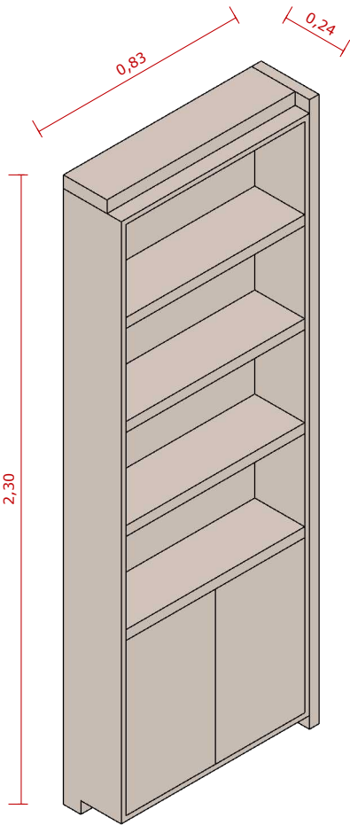
VISTA ISOMÉTRICA ESC. 1:20
