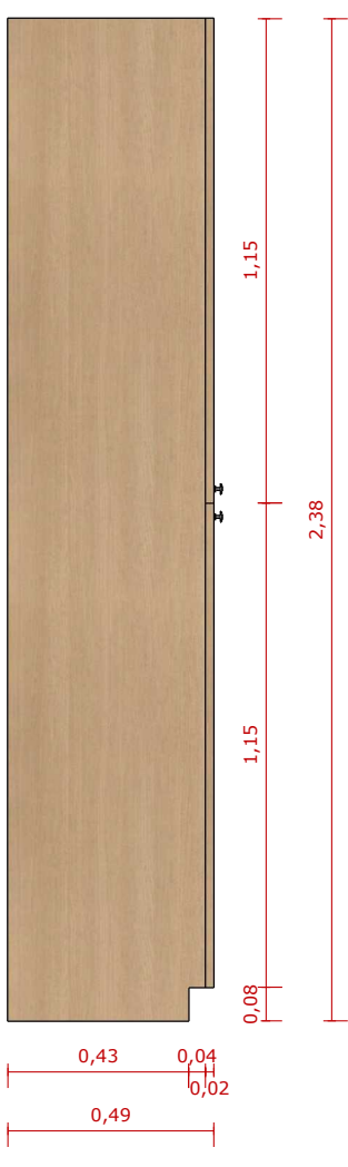
VISTA LATERAL ESC. 1:20
