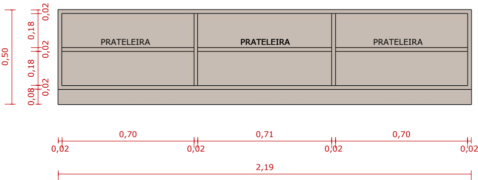
VISTA INTERNA ESC. 1:20
