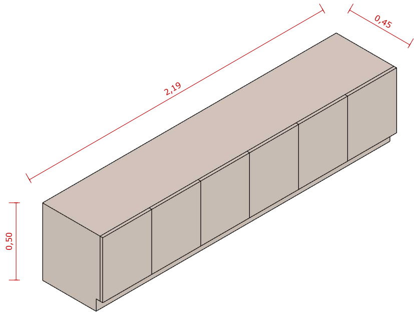
VISTA ISOMÉTRICA ESC. 1:20
