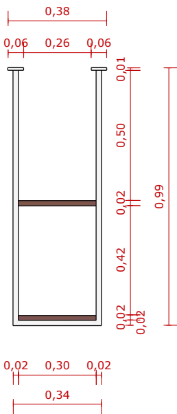
VISTA LATERAL ESC. 1:20
