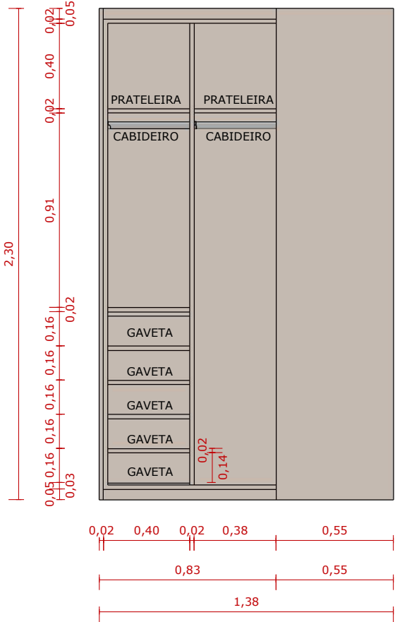
VISTA LATERAL INTERNA ESC. 1:25
