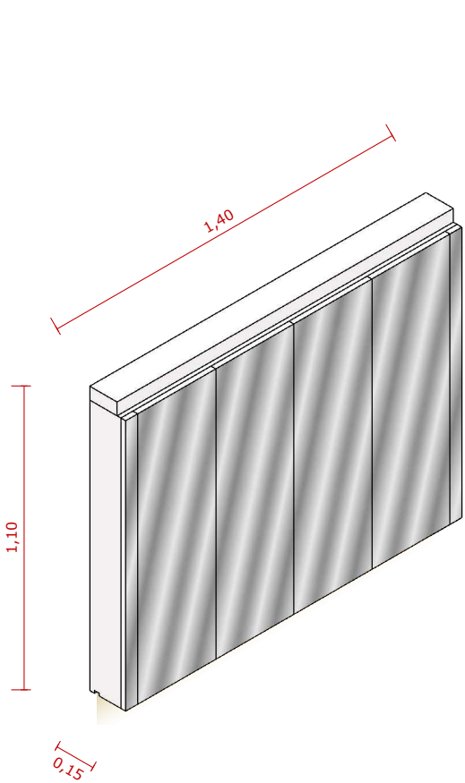
VISTA ISOMÉTRICA ESC. 1:20
