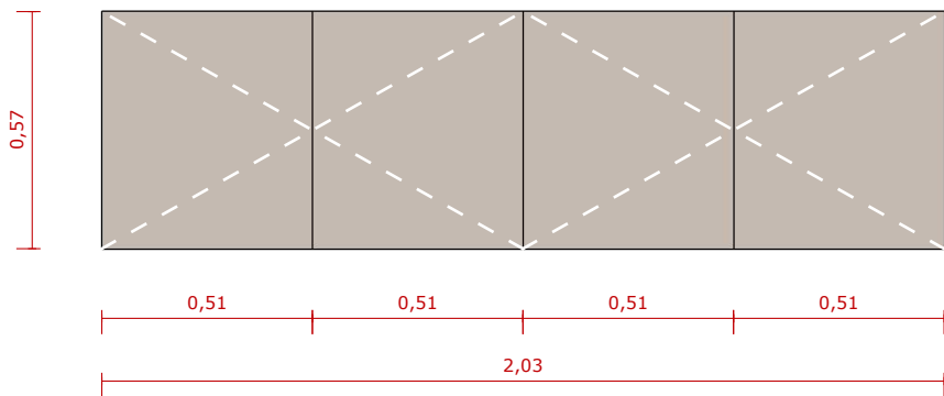
VISTA FRONTAL ESC. 1:20
