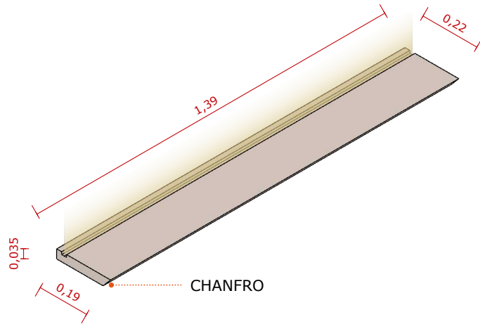
VISTA ISOMÉTRICA ESC. 1:15
