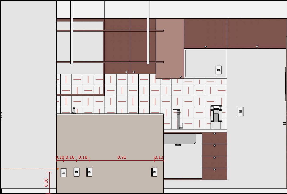
VISTA B ESC. 1:25
