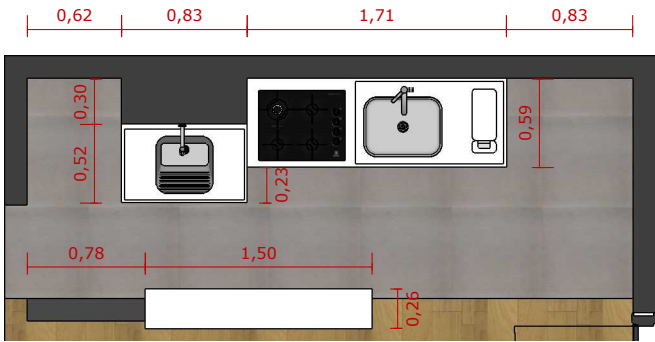
PLANTA COZINHA ESC. 1:50
