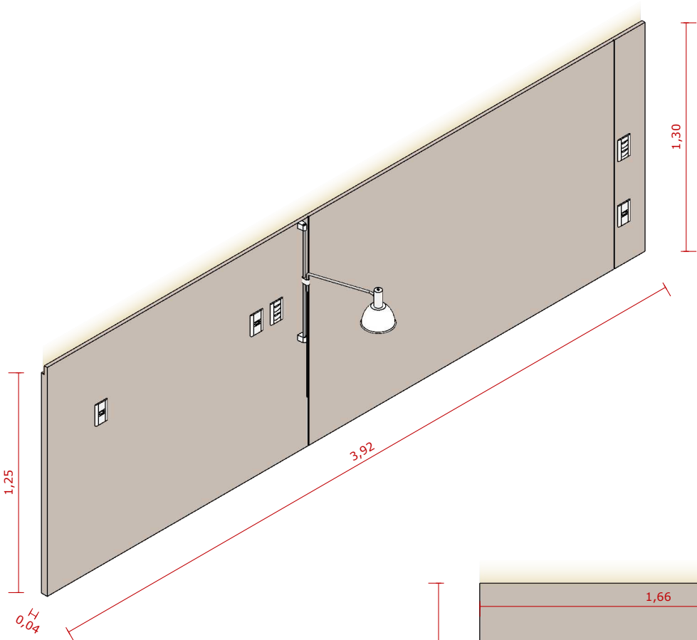
VISTA ISOMÉTRICA ESC. 1:25
