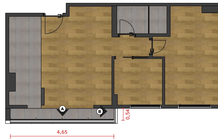
PLANTA ESC. 1:50
