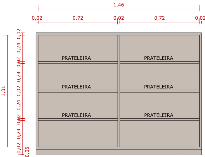
VISTA INTERNA ESC. 1:20
