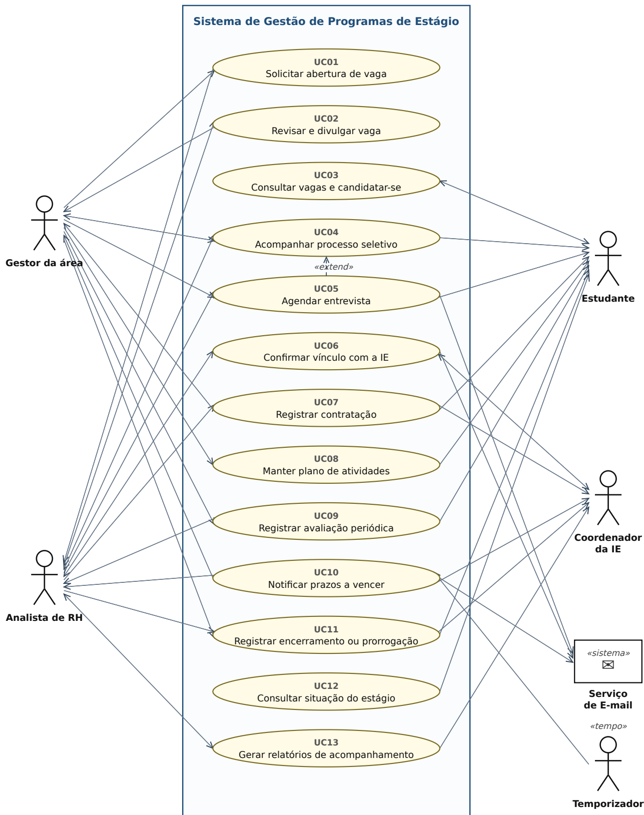
Figura 1 — Casos de uso requeridos (UC01-UC13)
