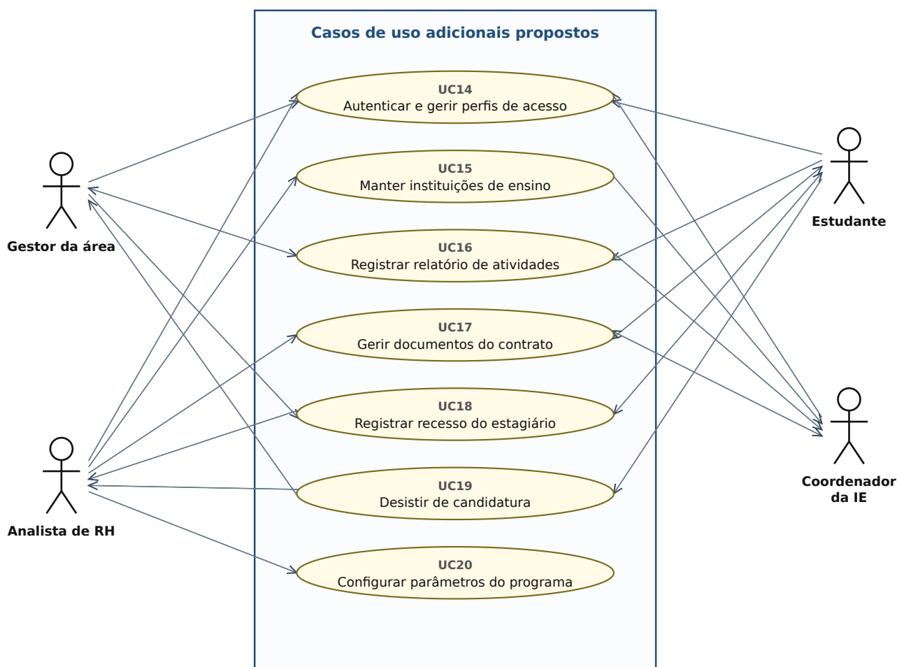
Figura 2 — Casos de uso adicionais propostos (UC14-UC20), com a mesma convenção de setas
