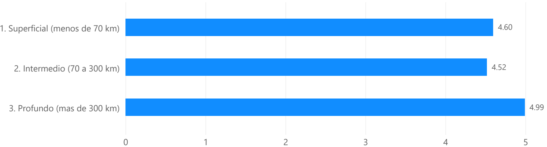
Magnitud Promedio por Rango de Profundidad
