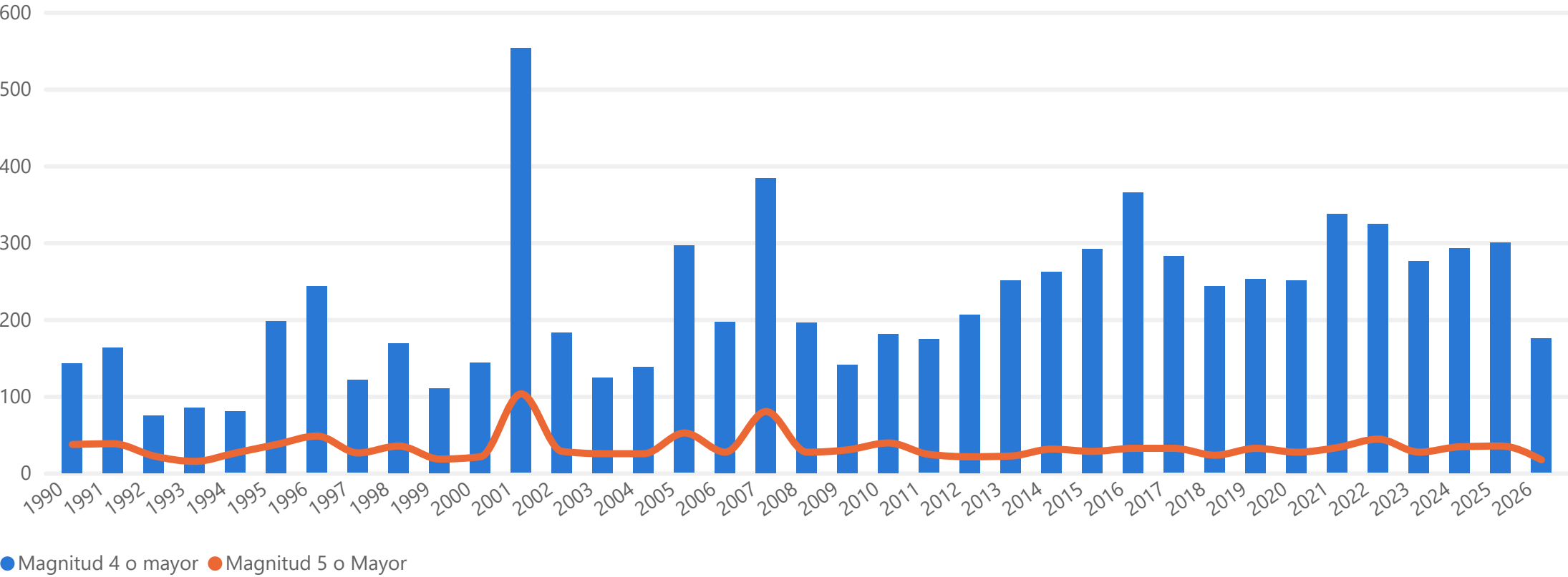
Detección Creciente, Sismicidad Estable
