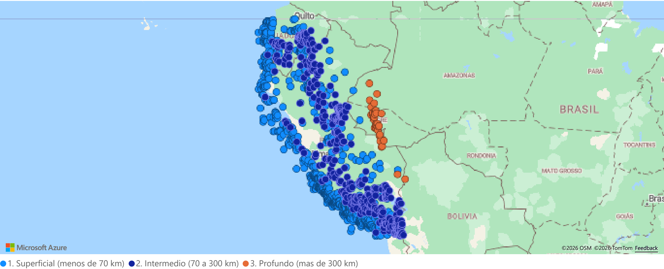
Epicentros de Magnitud 5 o Mayor, por Profundidad
