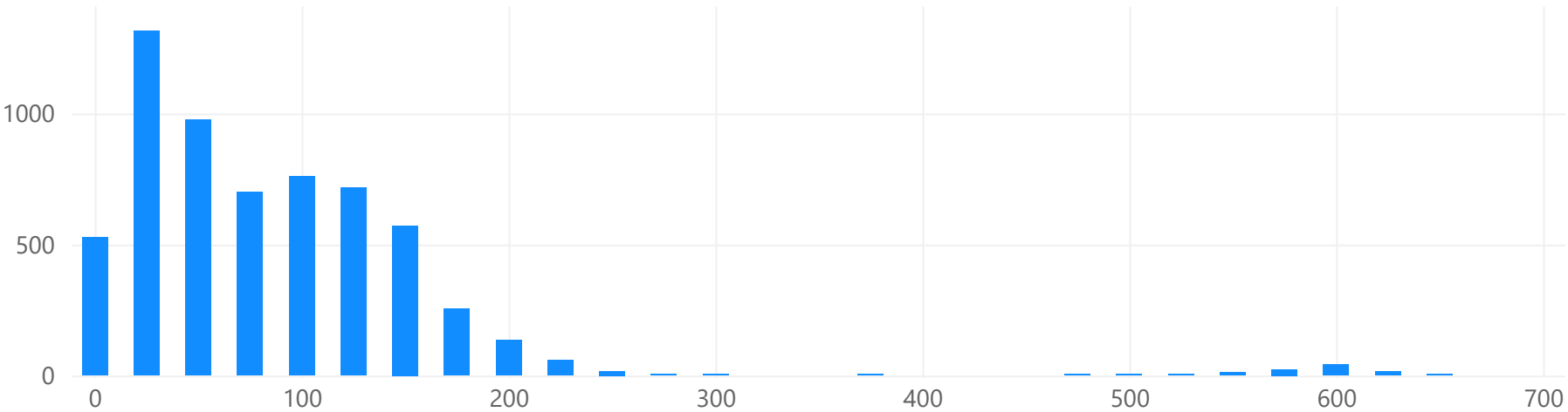
Distribución de Profundidades
