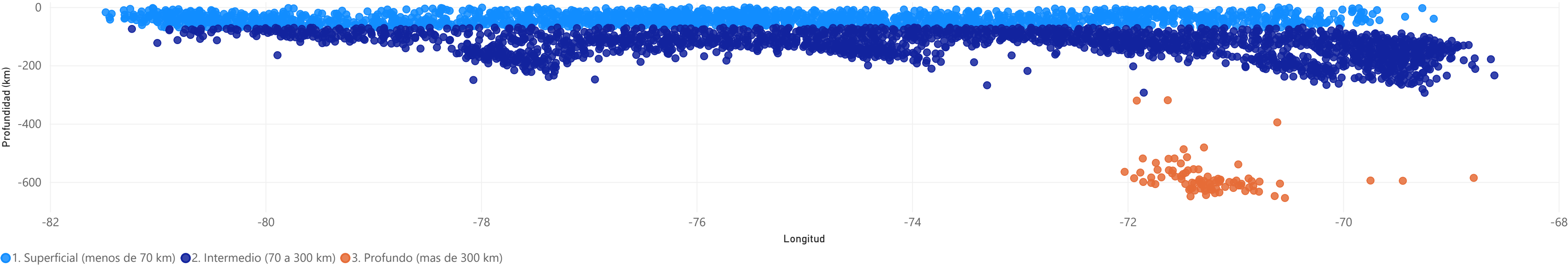
Corte transversal: la placa de Nazca bajo el Perú
