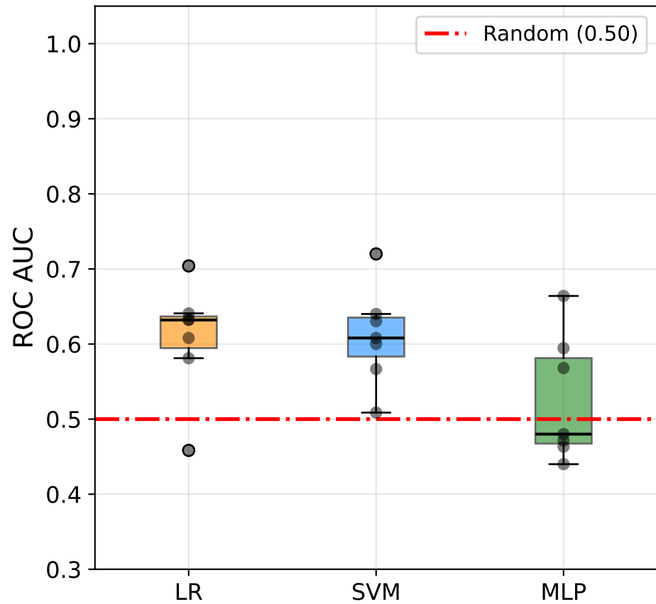
Final Model ROC AUC
