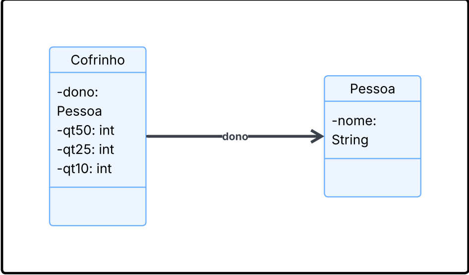
Diagrama de Classes — Cofrinho
