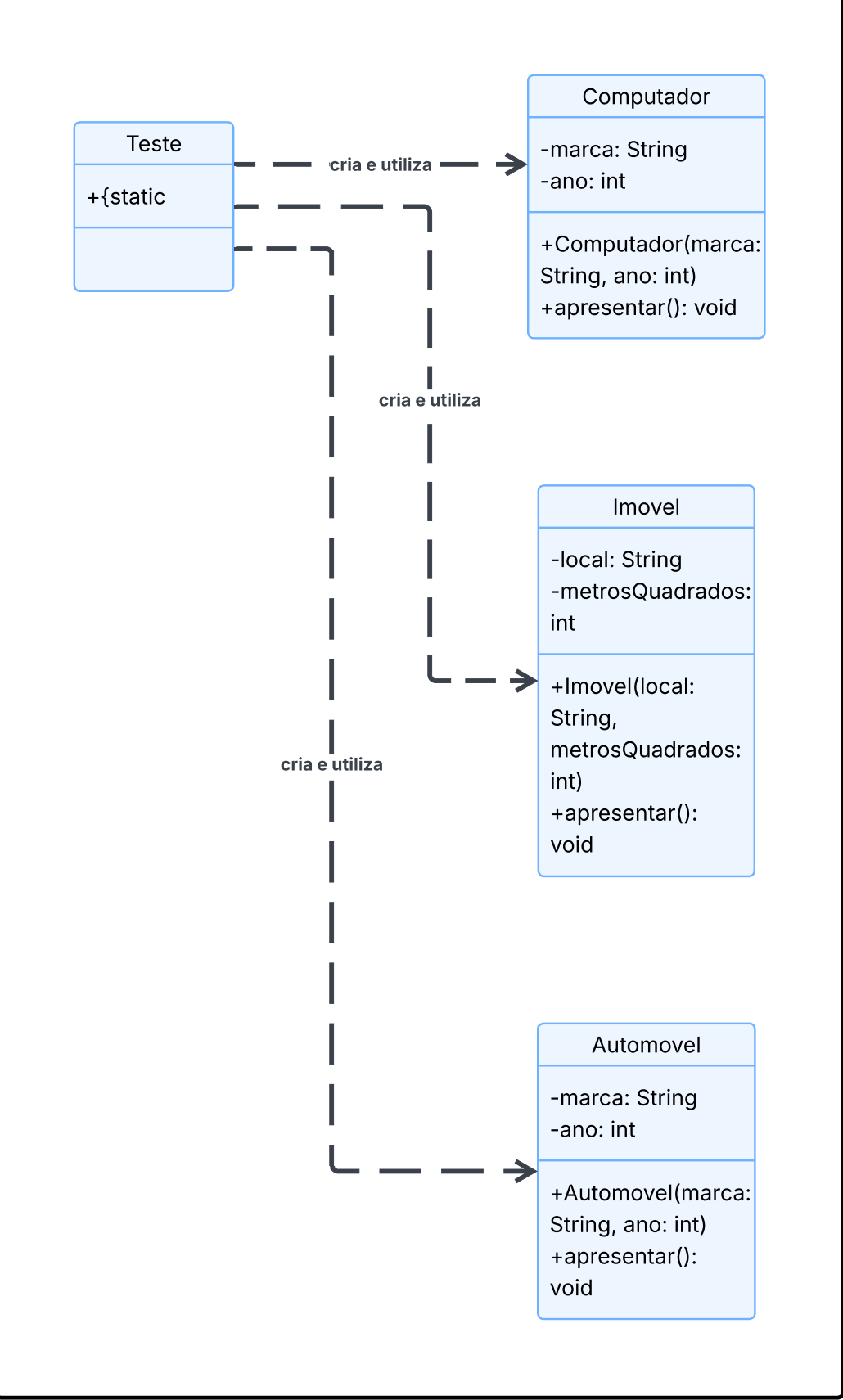
Diagrama de Classes — Sistema de Teste
