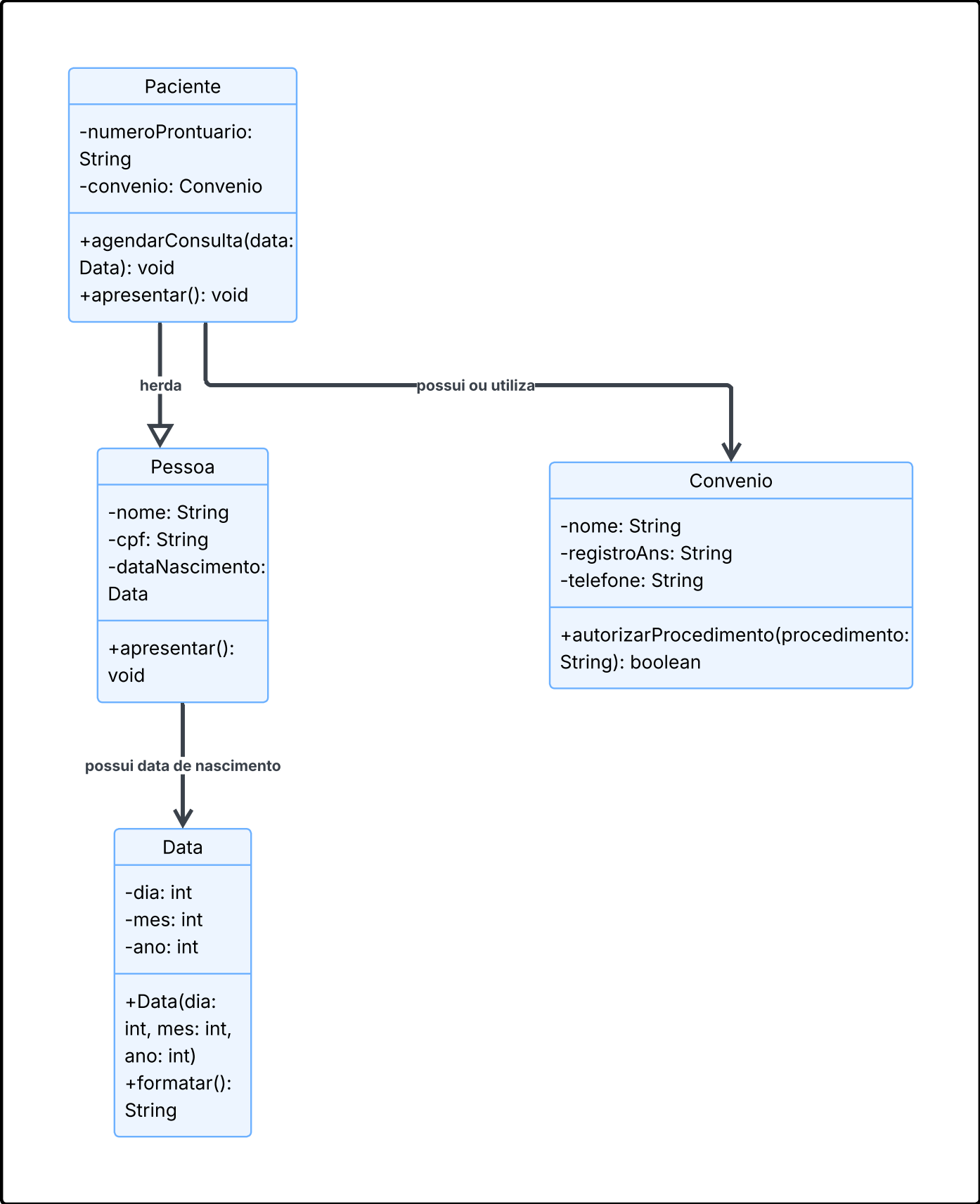
Diagrama de Classes — Pessoa, Paciente e Convênio
