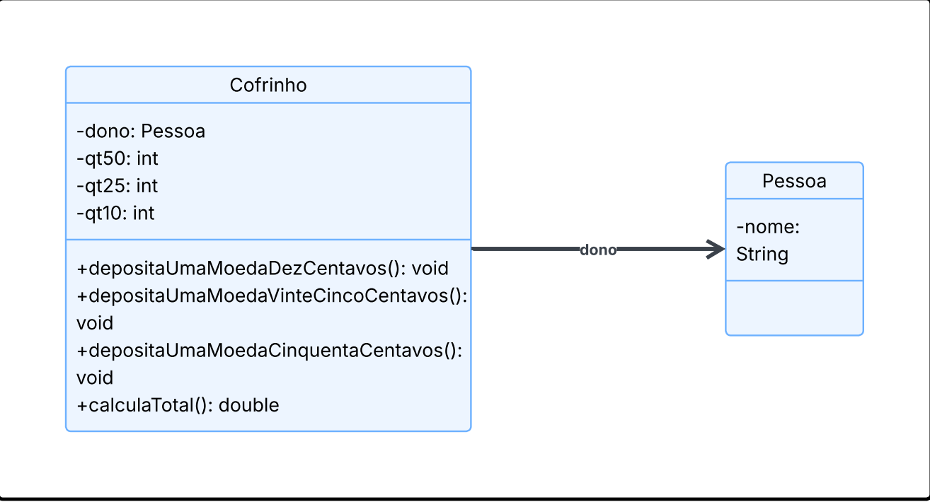
Diagrama de Classes — Cofrinho
