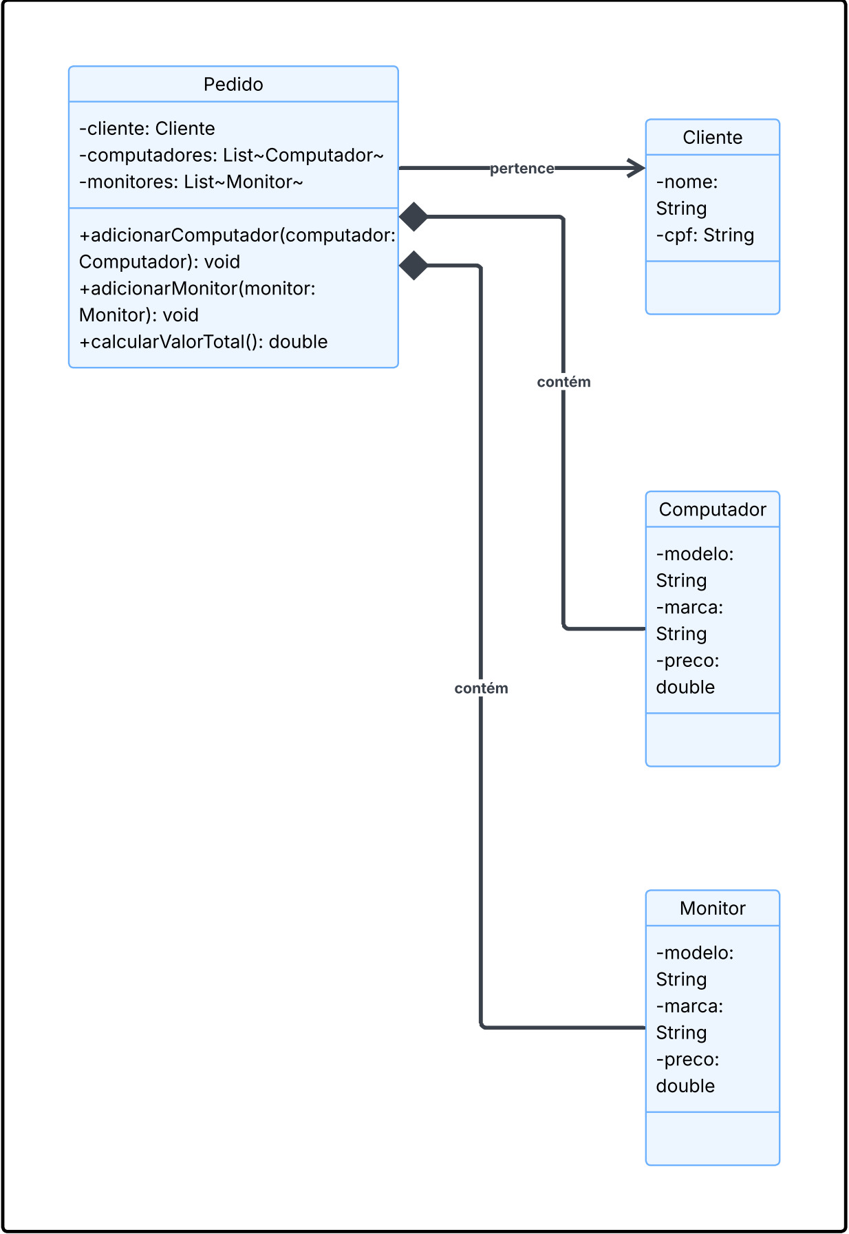
Diagrama de Classes — Pedido de Computadores
