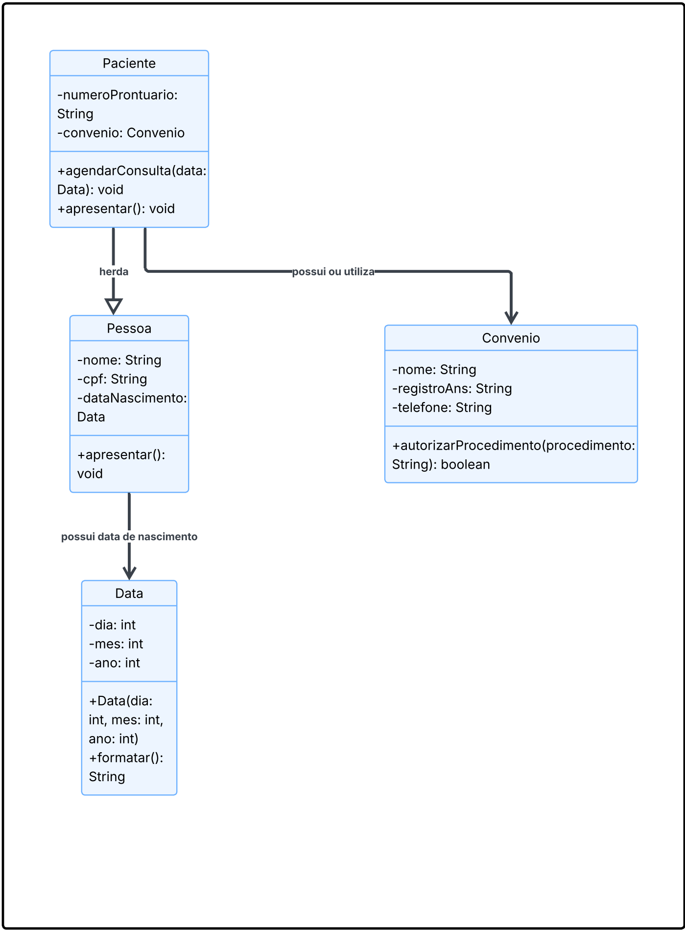
Diagrama de Classes — Pessoa, Paciente e Convênio
