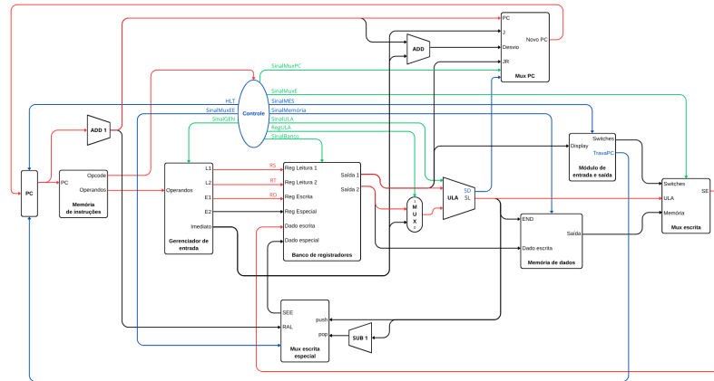
Figura 3 – Caminho de dados - Formato 1 (add, sub, mul, div, and, or, xnor)
