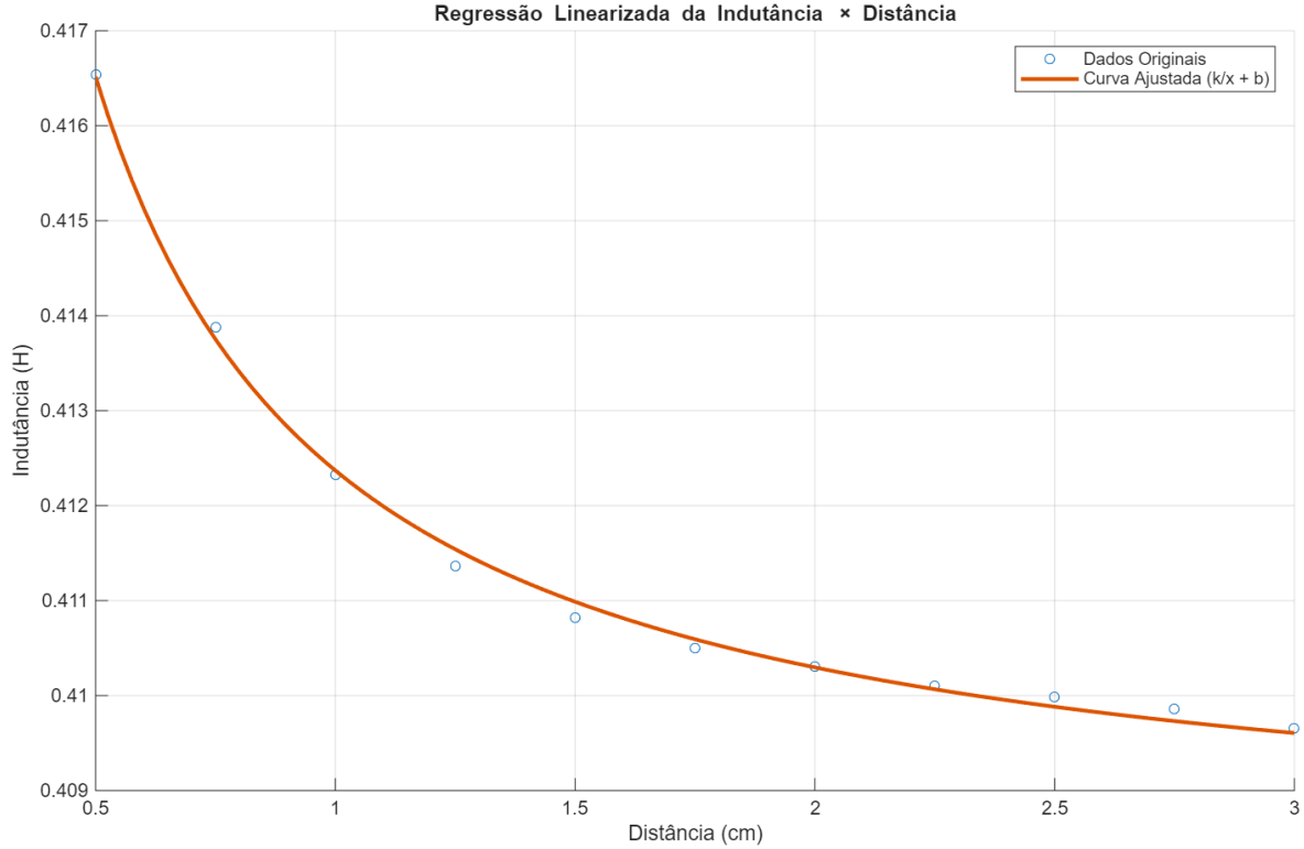
Figura 3.5: Comparação entre os valores de indutância obtidos no FEMM e a curva ajustada pelo modelo L(x) = k_L/x + L_b .
