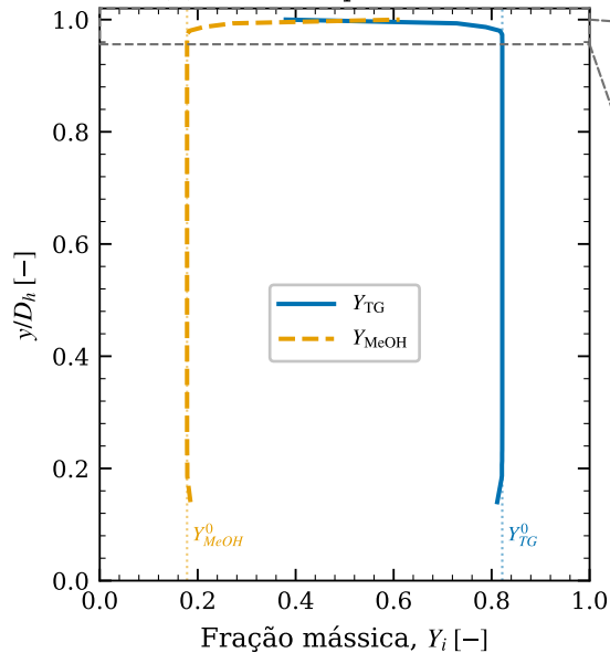
(a) Perfil completo — x/L=1
