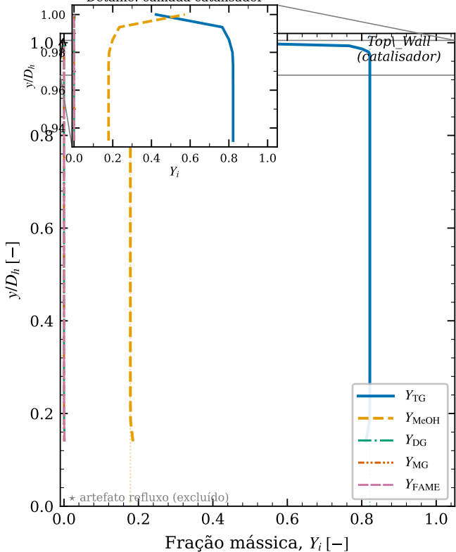
Detalhe: camada catalisador
