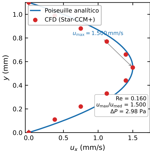
(a) Perfil de velocidade — saída ( x = L )
