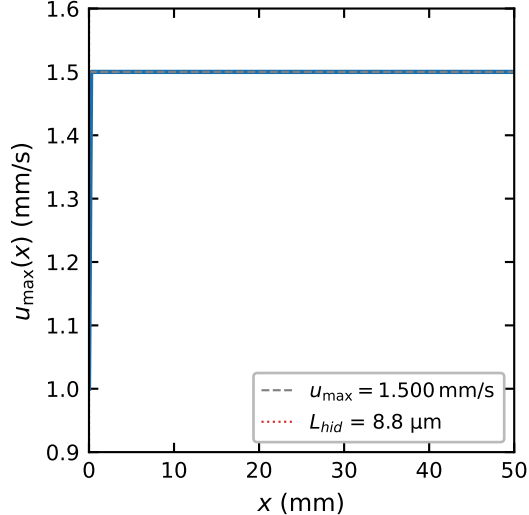
(b) Desenvolvimento axial — u_{\max}(x)
