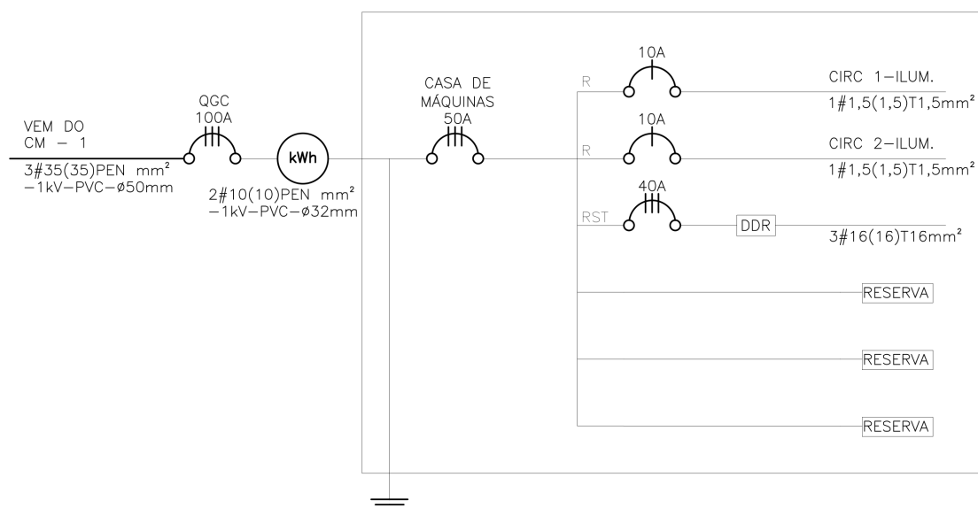
Figura 7 – Quadro da casa de máquinas.
