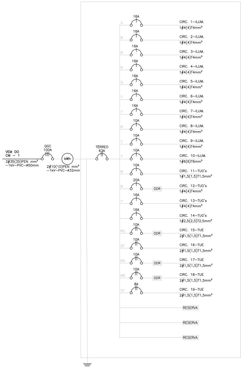
Figura 10 – Unifilar do T rreo.
