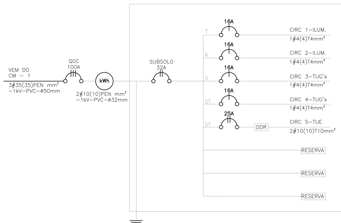
Figura 8 – Unifilar do Subsolo.
