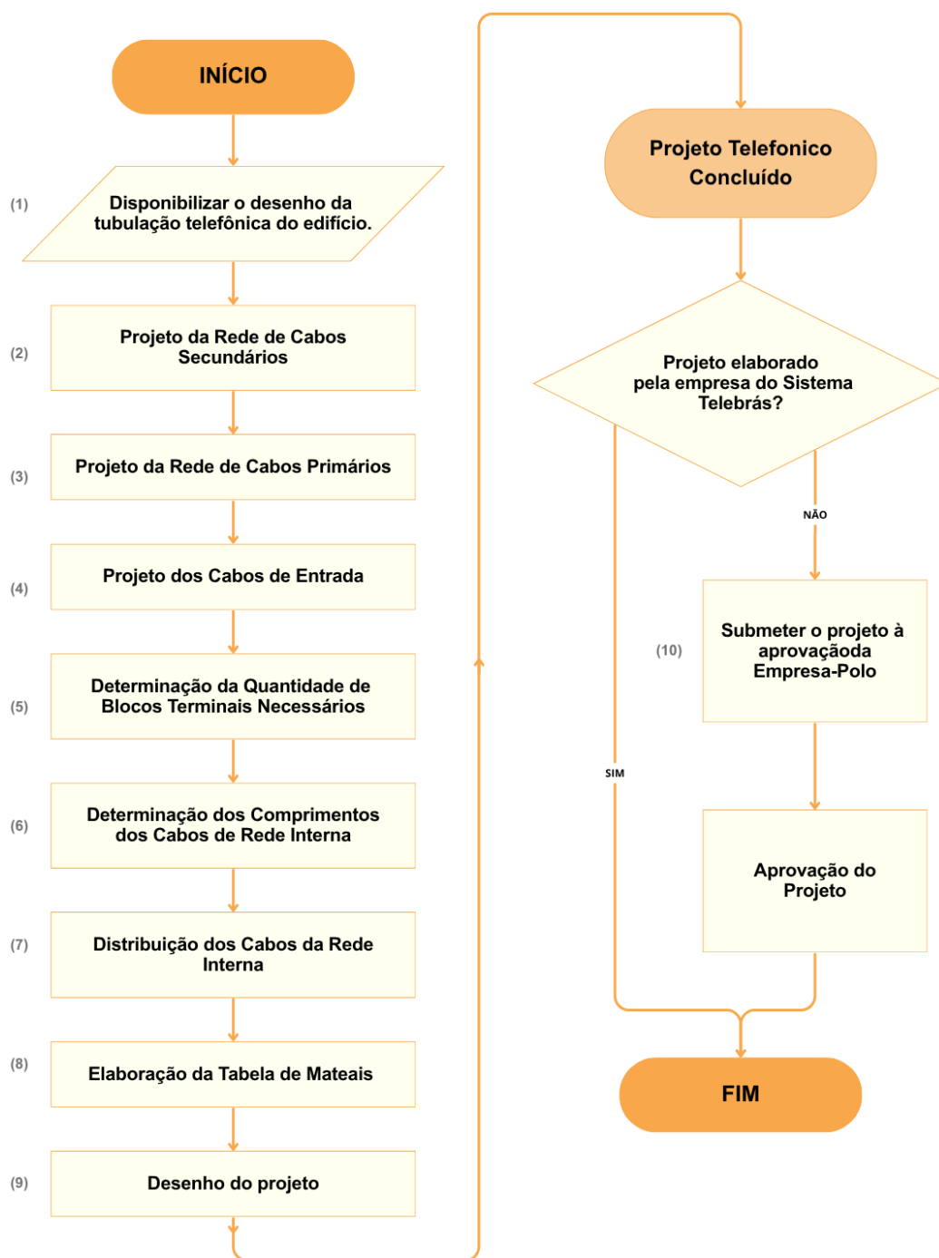
Figura 13 – Fluxograma da sequência de passos para o dimensionamento de um projeto telefônico.
