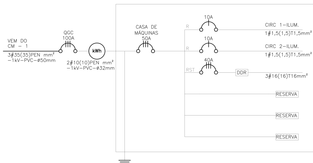
Figura 12 – Unifilar do Máquinas.
