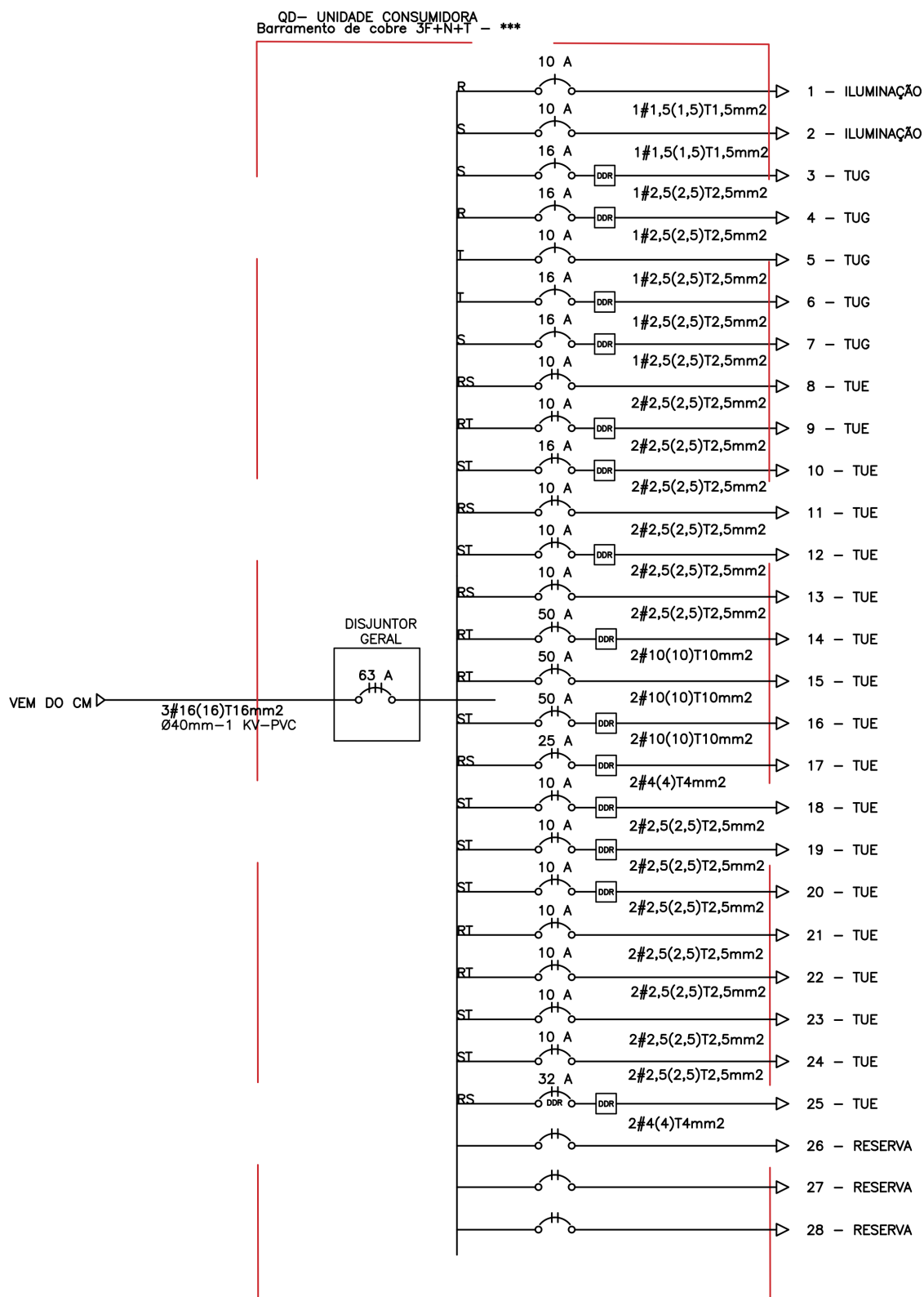
Figura 11 – Diagrama Unifilar dos Apartamentos.
