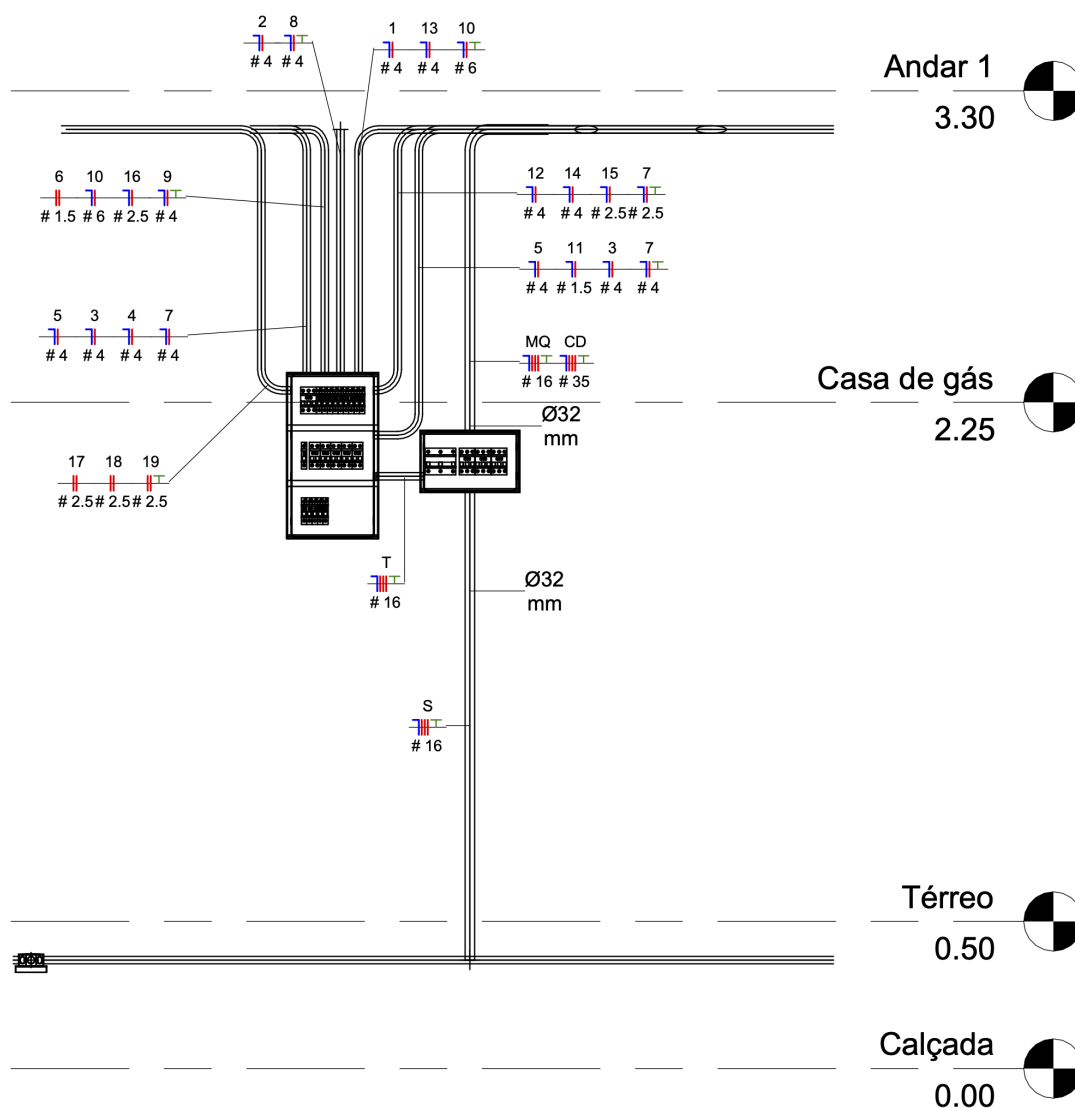
Figura 5 – QGC e quadro do térreo.
