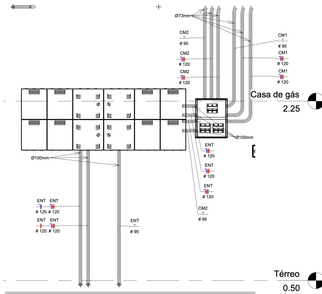
Figura 4 – Quadro da Caixa seccionadora e QGBT.
