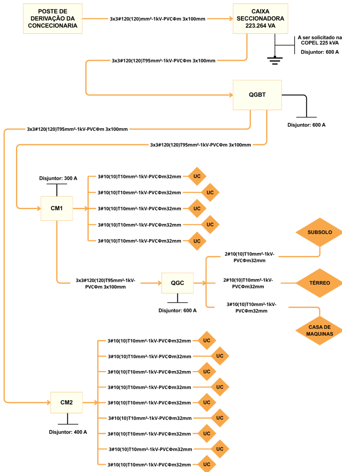
Figura 2 – Fluxograma do projeto elétrico.
