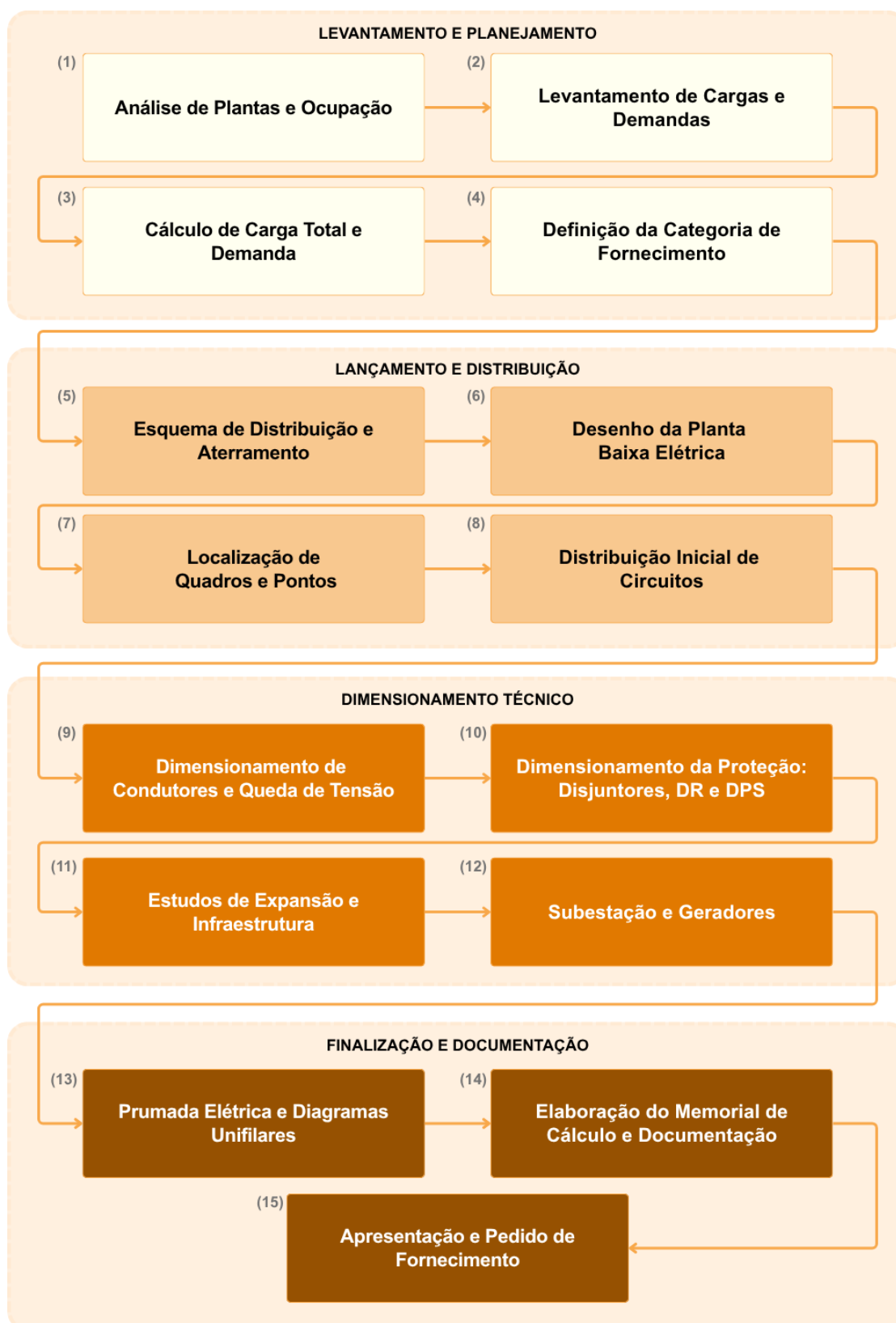
Figura 1 – Fluxograma do projeto elétrico.
