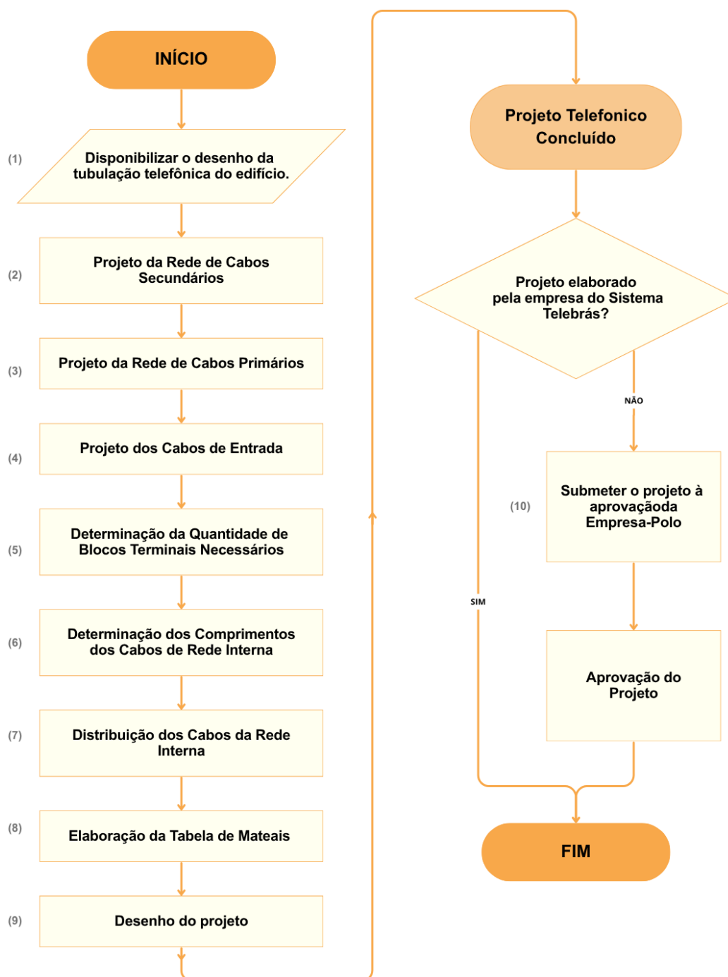
Figura 3 – Fluxograma da sequência de passos para o dimensionamento de um projeto telefônico.
