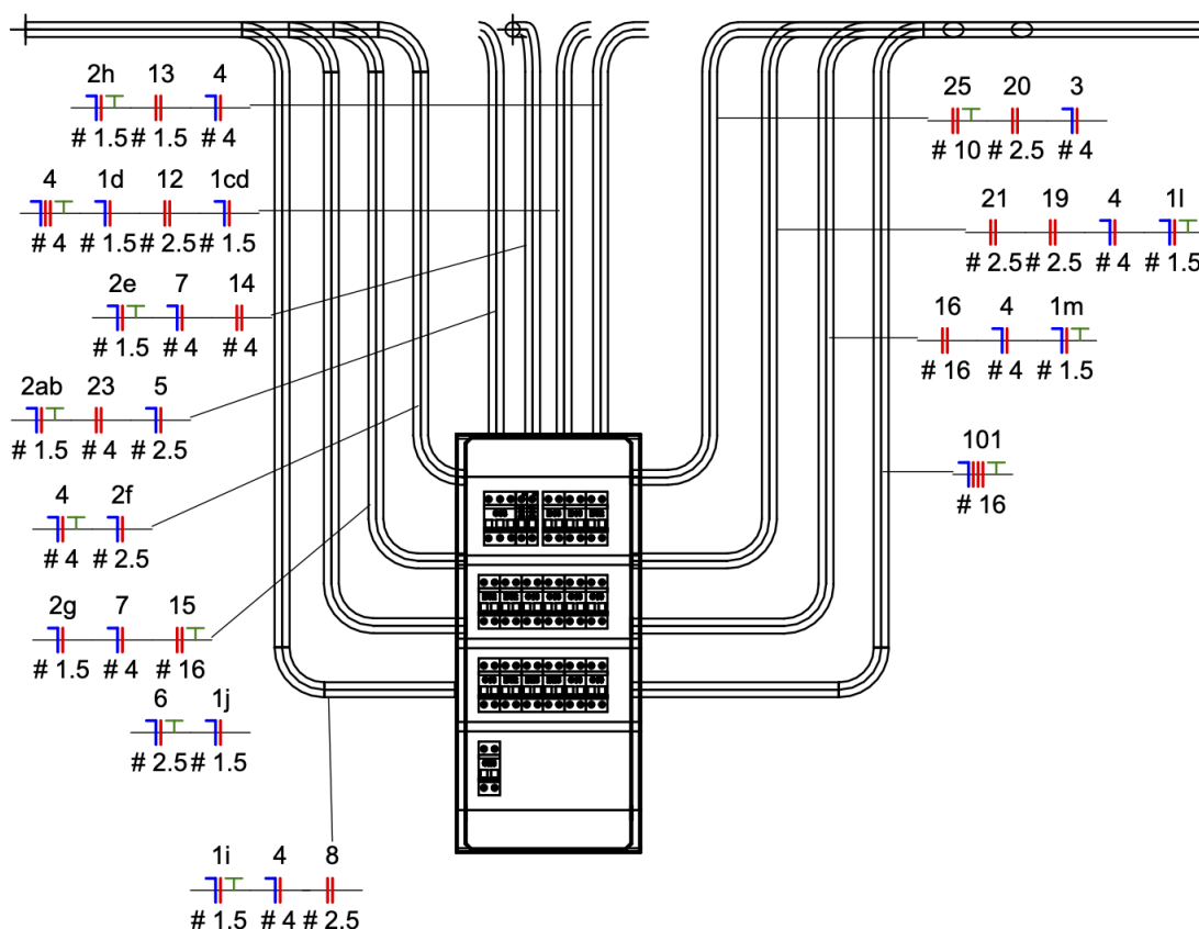
Figura 8 – Quadro do apartamento.
