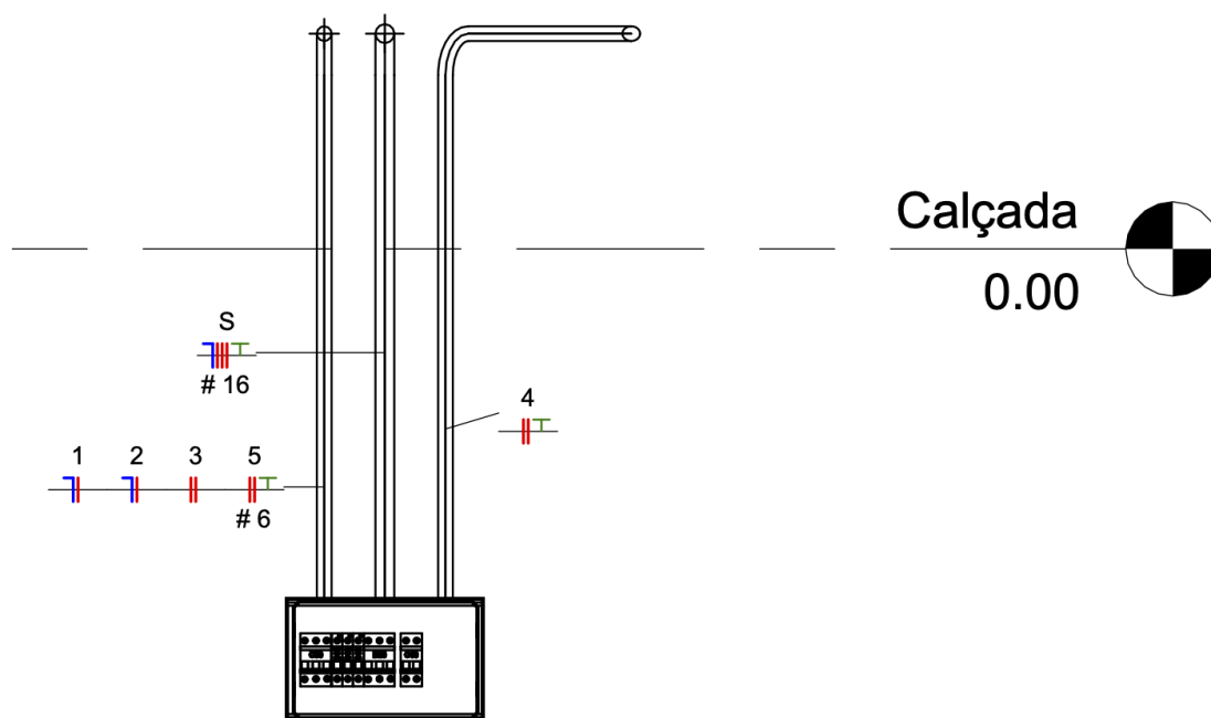
Figura 5 – Quadro do Subsolo.
