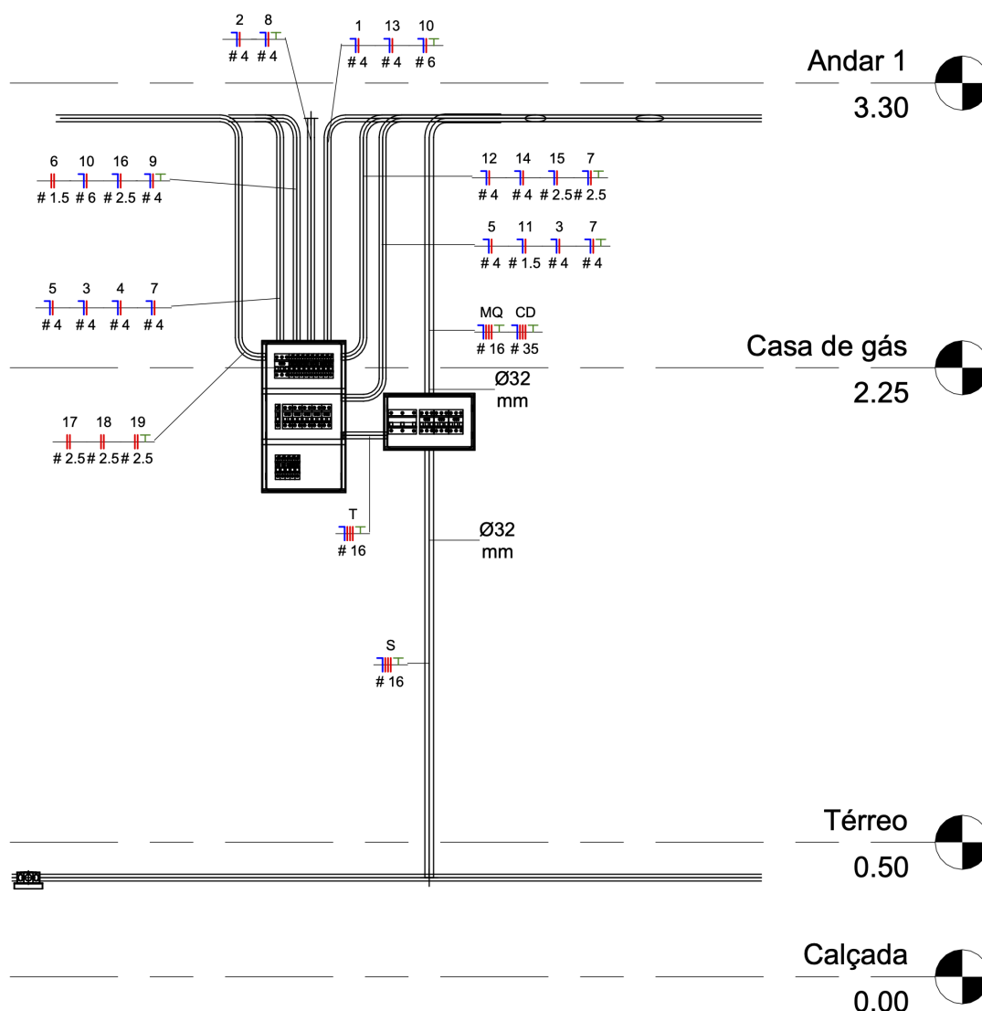
Figura 7 – QGC e quadro do térreo.
