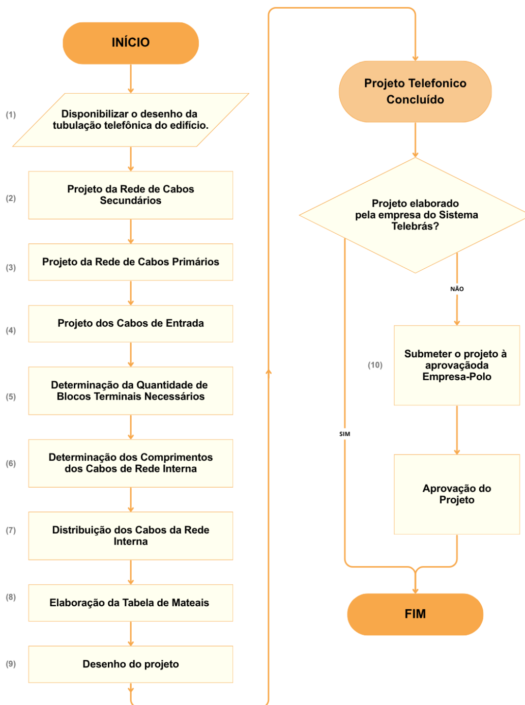
Figura 19 – Fluxograma da sequência de passos para o dimensionamento de um projeto telefônico.
