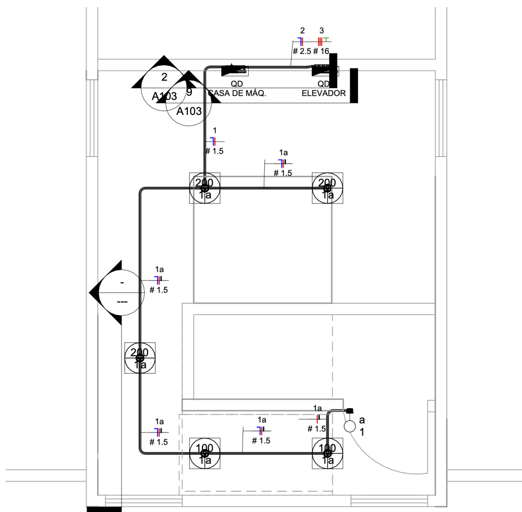
Figura 18 – Planta de Instalação Eletrica da Casa de Maquinas.
