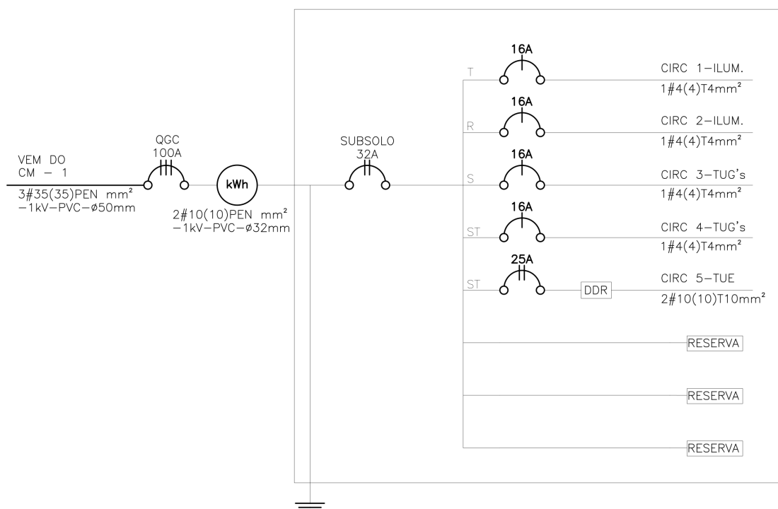
Figura 10 – Unifilar do Subsolo.
