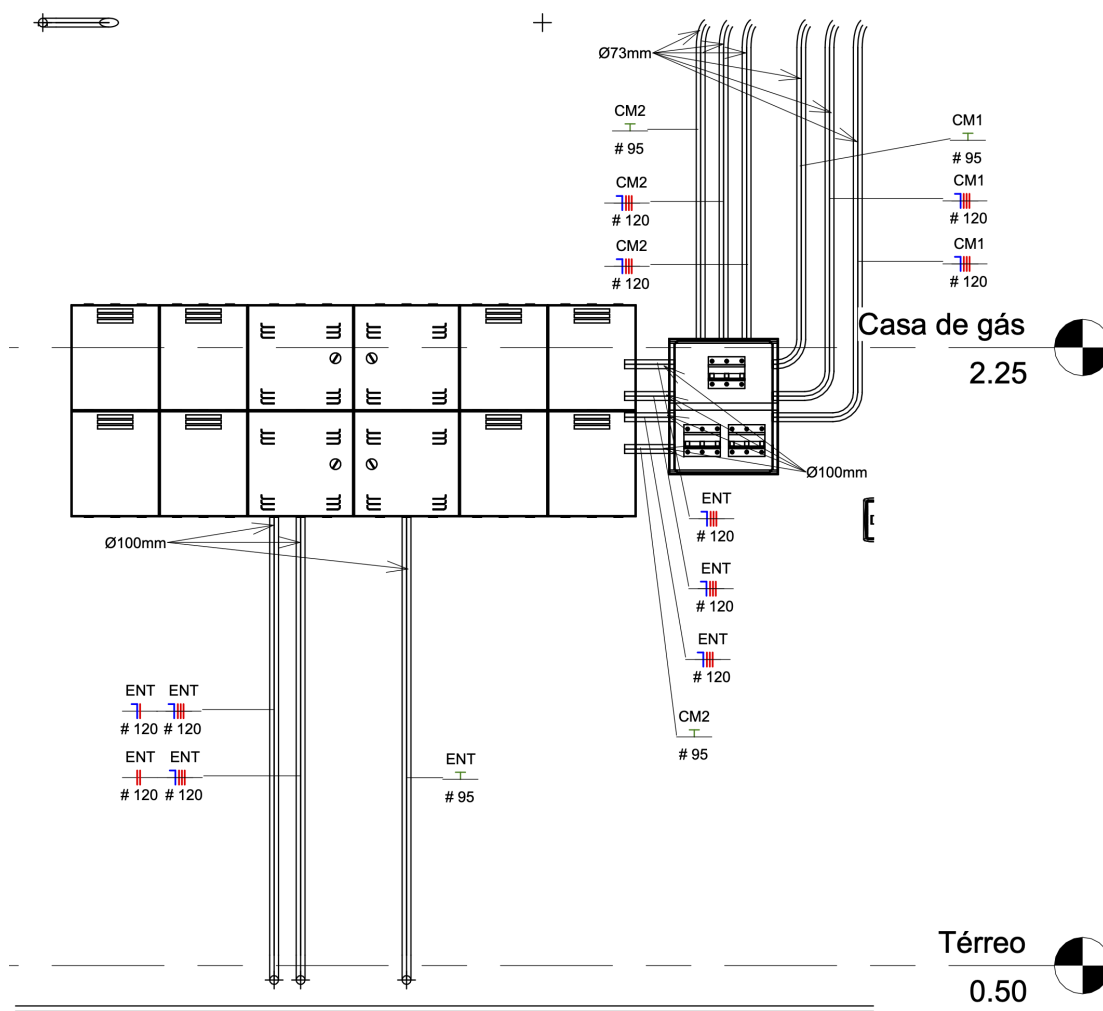
Figura 6 – Quadro da Caixa seccionadora e QGBT.
