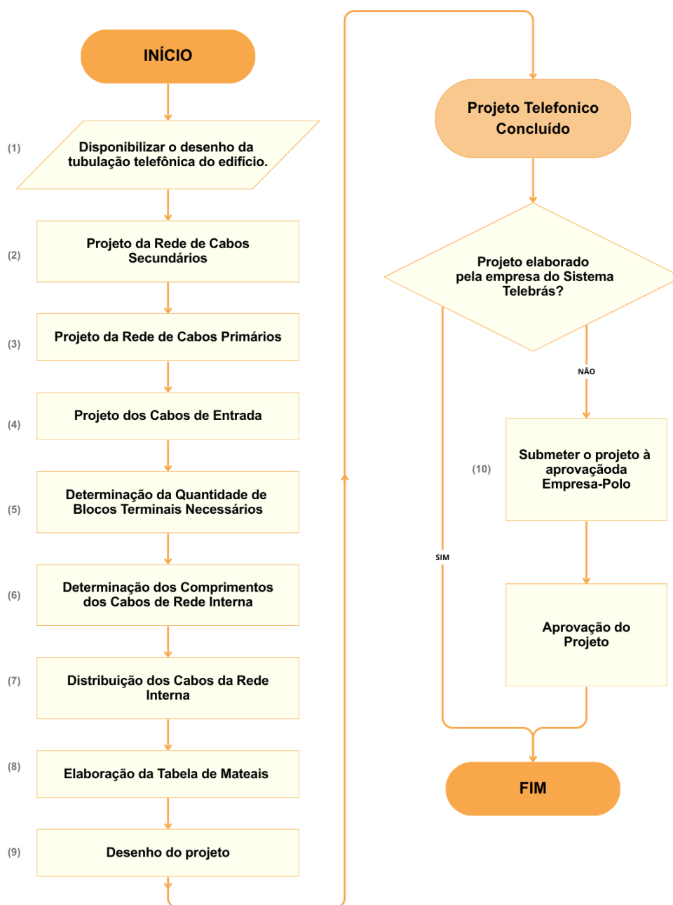
Figura 2 – Fluxograma da sequência de passos para o dimensionamento de um projeto telefônico.
