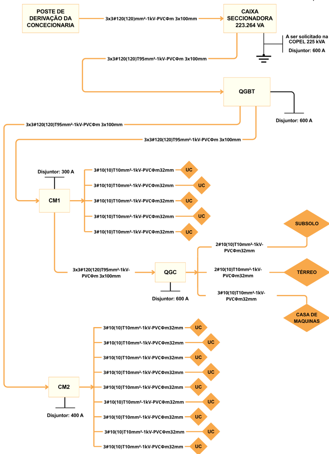
Figura 1 – Fluxograma do projeto elétrico.
