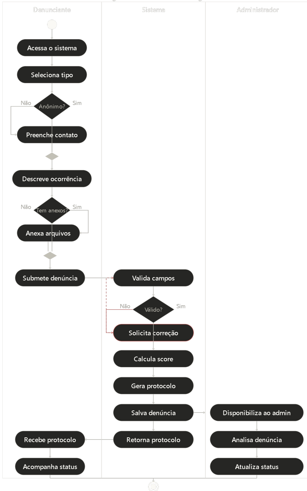
Diagrama de Atividades — Protege+
