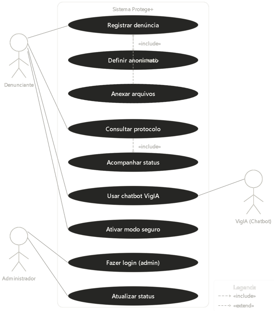
Diagrama de Casos de Uso — Protege+
