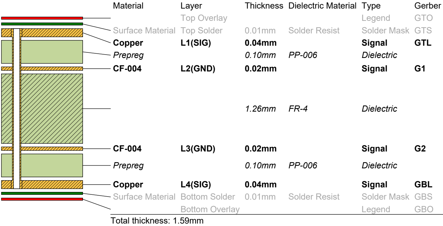
Layer Stack Legend
