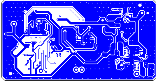
L4(SIG) (Scale 1:1)
