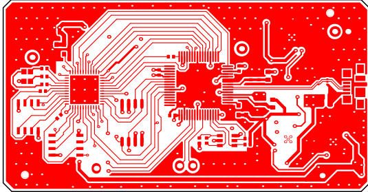
L1(SIG) (Scale 1:1)
