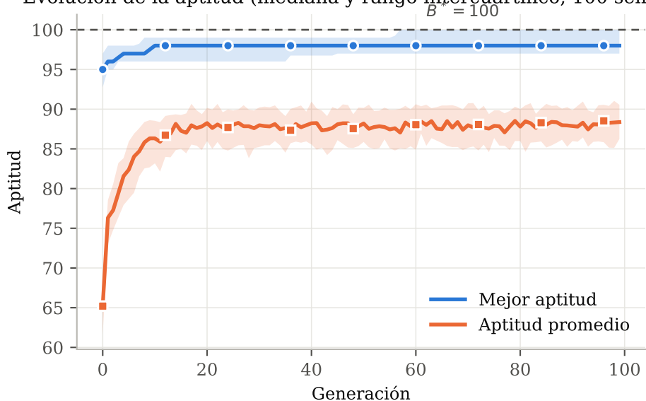
Evolución de la aptitud (mediana y rango intercuartílico, 100 semillas)
