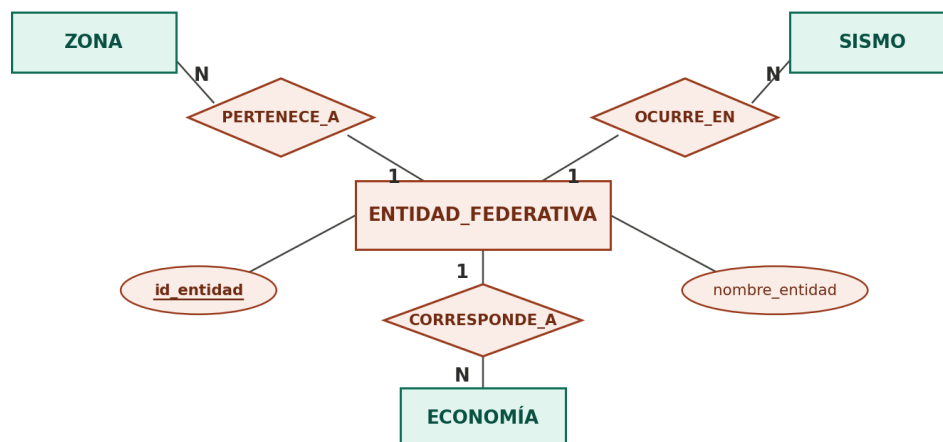
Figura 1. Nueva entidad ENTIDAD_FEDERATIVA y sus relaciones con ZONA, SISMO y ECONOMÍA.
